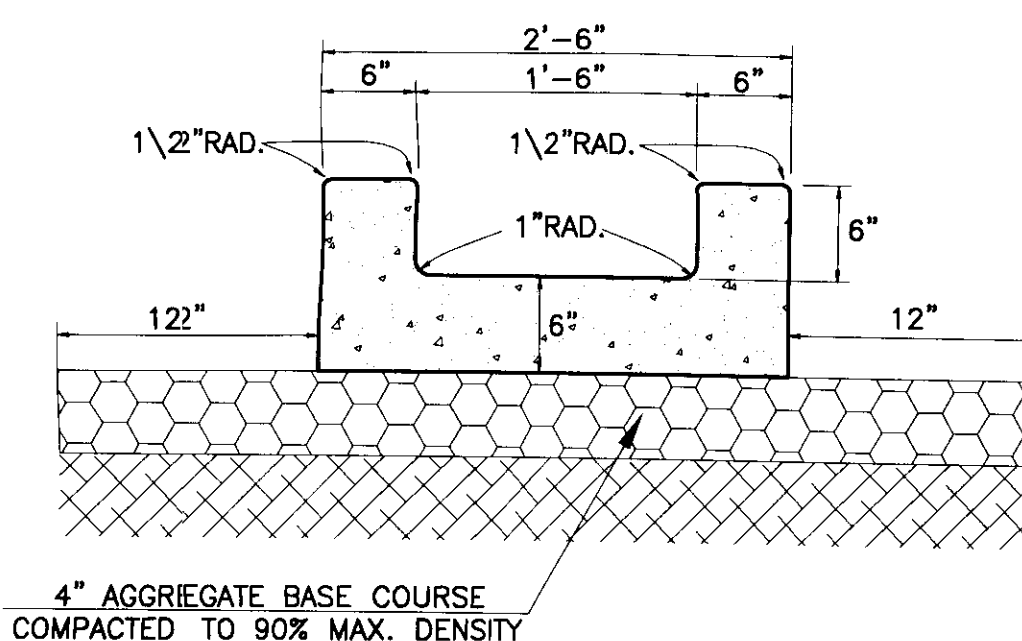
18' CONCRETE CHANNEL DETAIL: ⑮ N.T.S.
