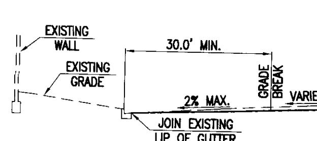
SECTION D-D: N.T.S.
