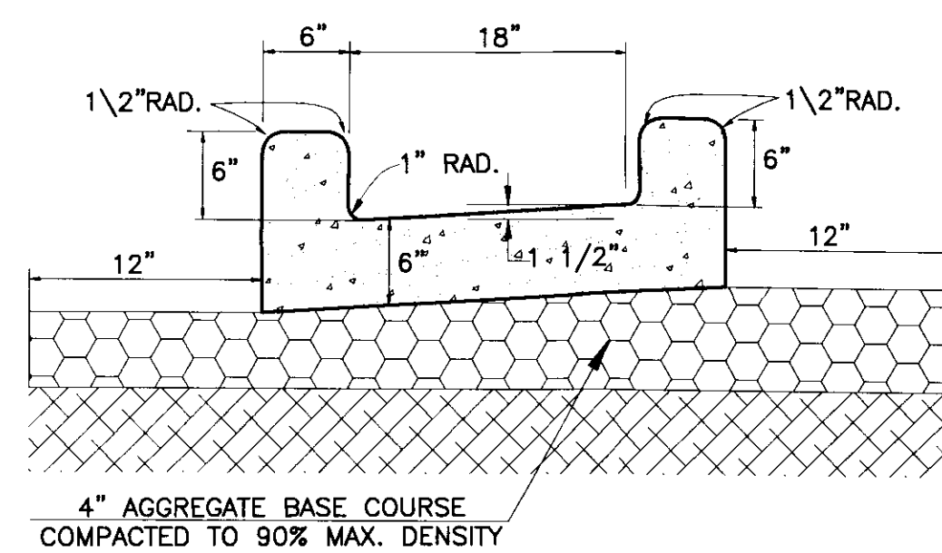
18' CONCRETE CHANNEL DETAIL: ⑪ N.T.S.
