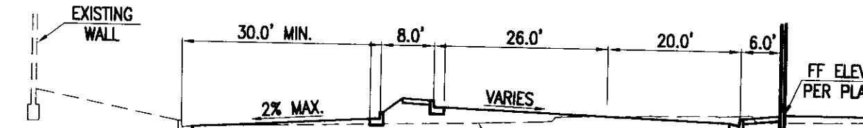
SECTION C-C: N.T.S.
