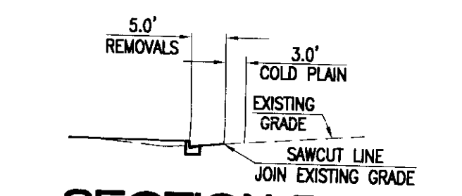
SECTION B-B: N.T.S.
