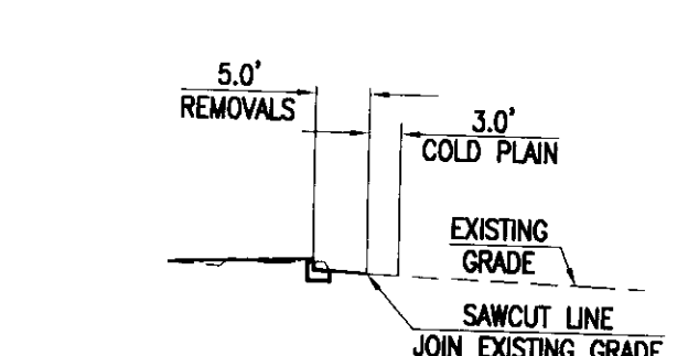
SECTION E-E: N.T.S.
