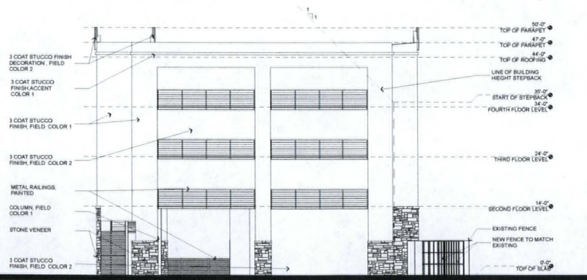
D1 NORTH ELEVATION
