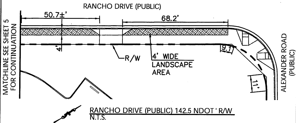
RANCHO DRIVE SECTION N.T.S.
