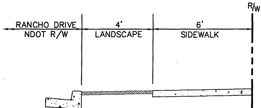
RANCHO DRIVE SECTION N.T.S.
