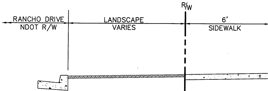
RANCHO DRIVE SECTION N.T.S.
