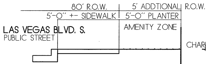
TYPICAL SECTION N.T.S.
