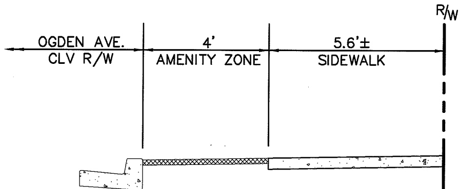
OGDEN AVENUE SECTION N.T.S.
