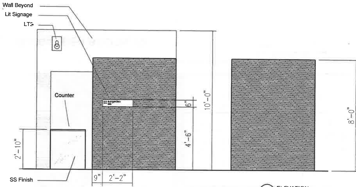
3.2 ELEVATION
