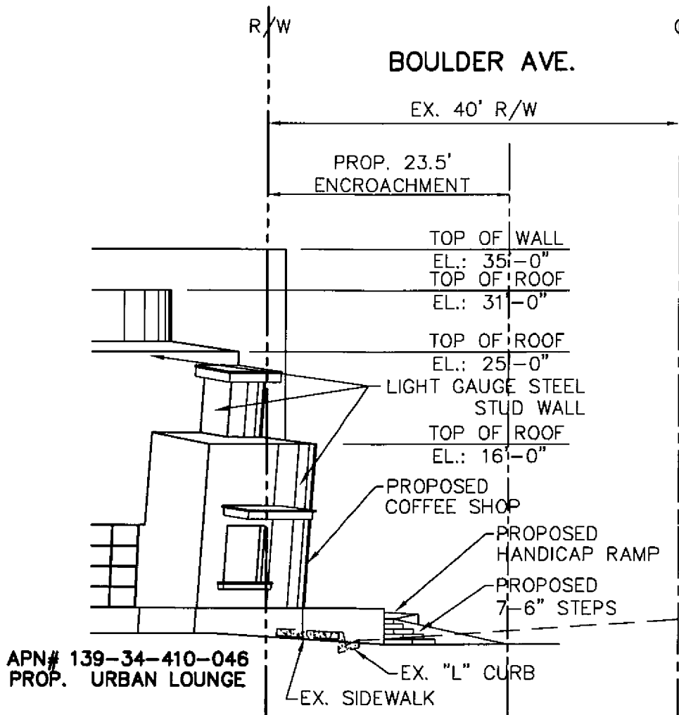
SECTION A SCALE: NTS
