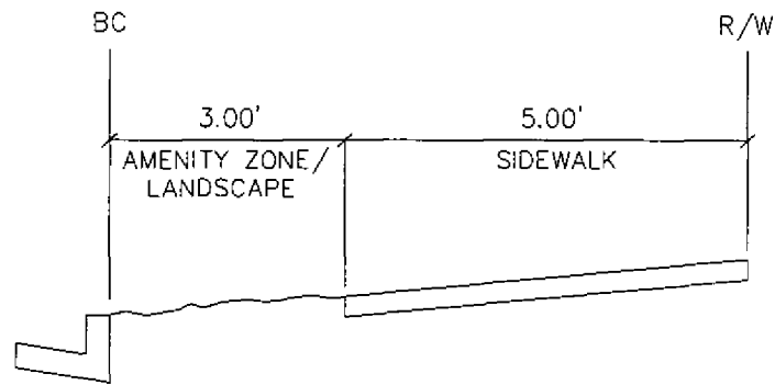
A 5 DEER SPRINGS WAY SECTION N.T.S
