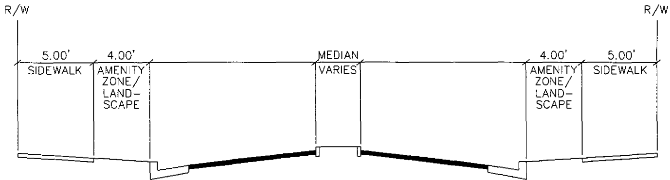
B 5 GRAND MONTECITO PARKWAY SECTION N.T.S
