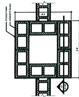
16) PILASTER DETAIL
