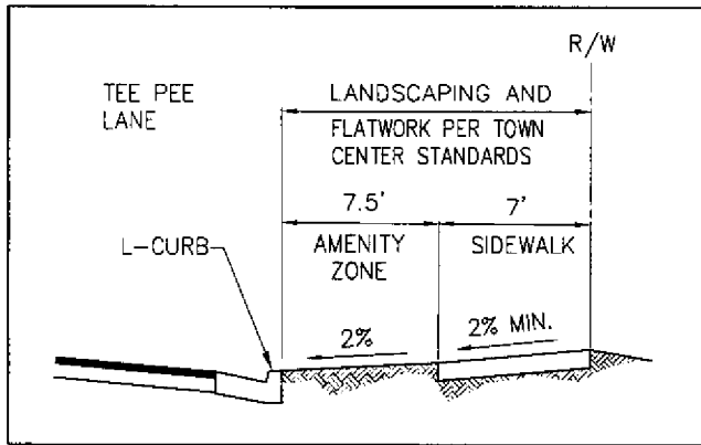
TYPICAL SECTION N.T.S.
