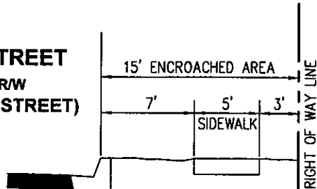
TYPICAL SECTION N.T.S.
