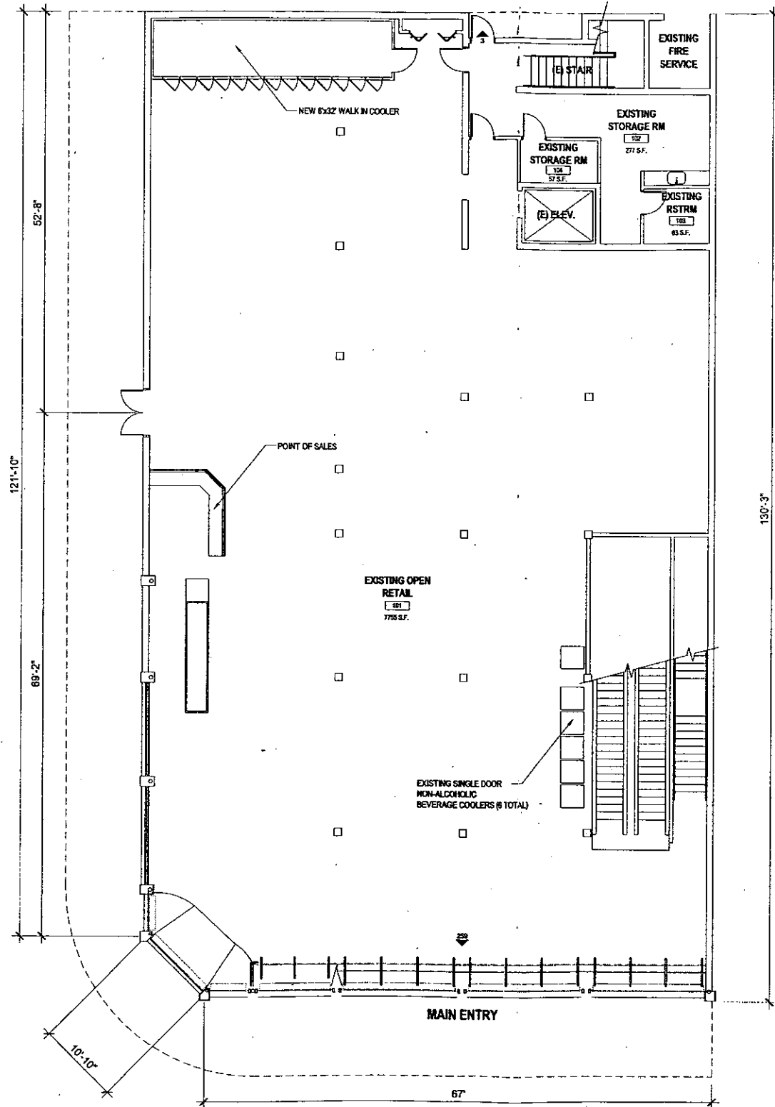
1 EXISTING FLOOR PLAN A1.00 SCALE: 1/8" = 1'-0"
