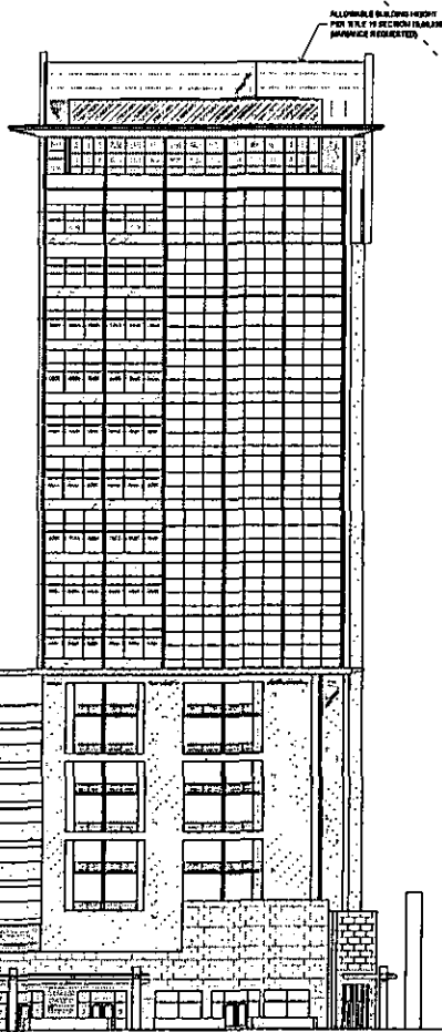
D1 EAST ELEVATION 1/8" = 1'-0"
