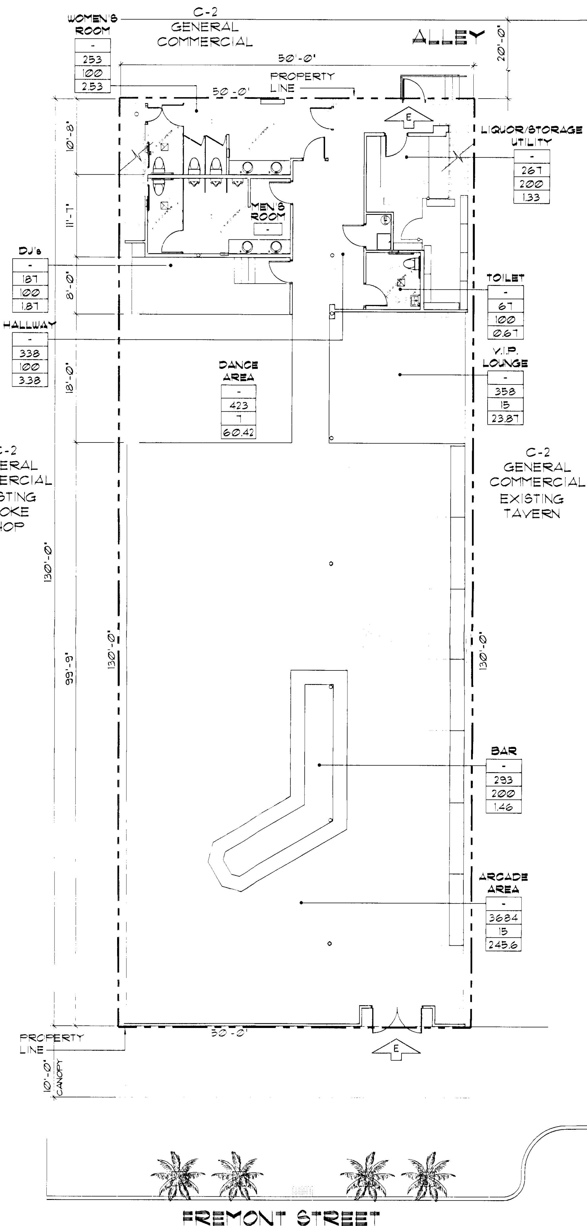
1 SITE / FLOOR PLAN A1.01 SCALE: 1/8" = 1'-0"
