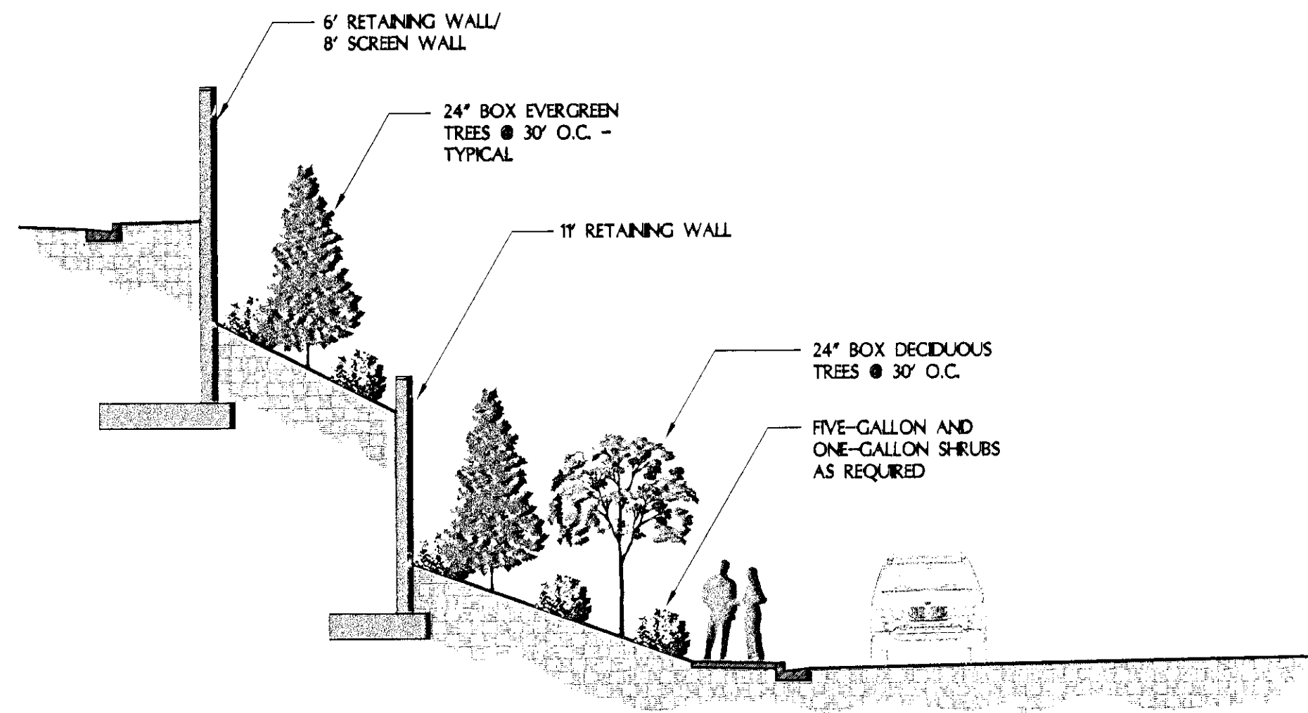
1 SITE SECTION SCALE: 1/8" = 1'-0"
