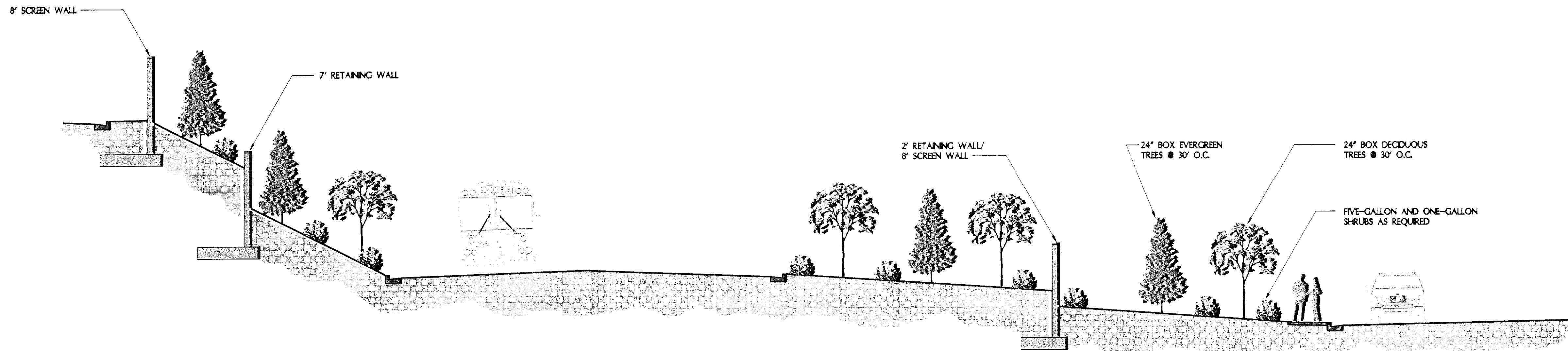
3 SITE SECTION SCALE: 1/8" = 1'-0"
