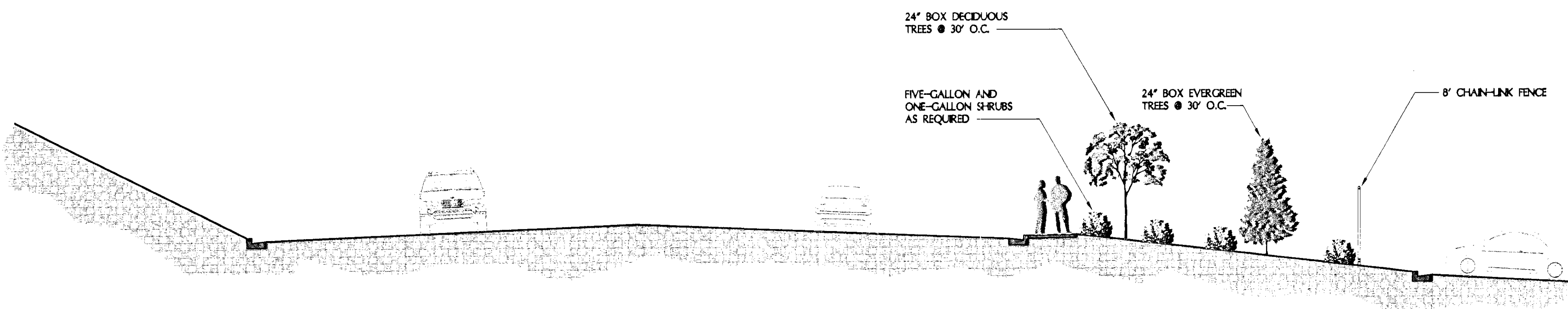
4 SITE SECTION SCALE: 1/8" = 1'-0"
