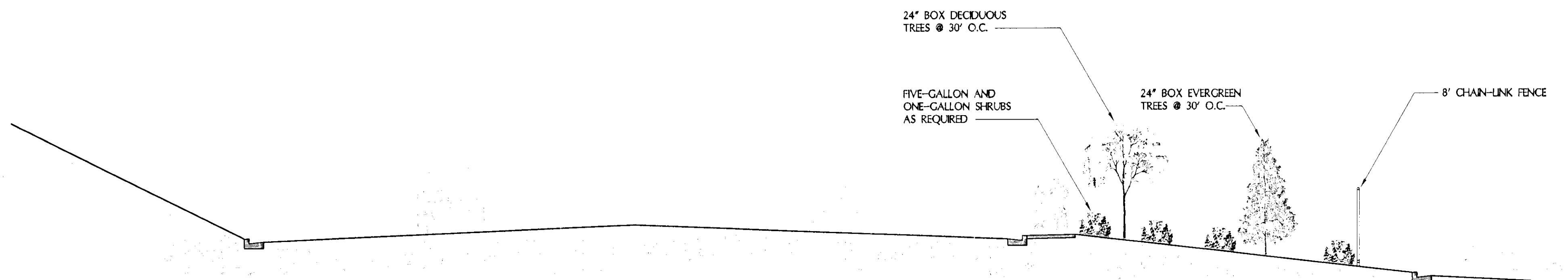
4 SITE SECTION SCALE: 1/8" = 1'-0"
