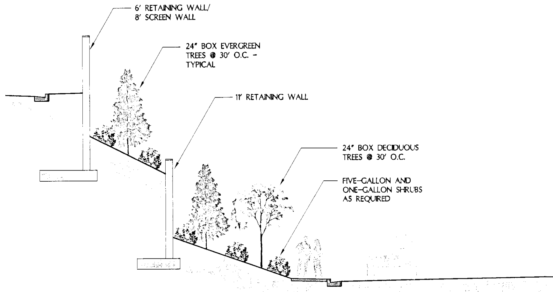
1 SITE SECTION SCALE: 1/8" = 1'-0"
