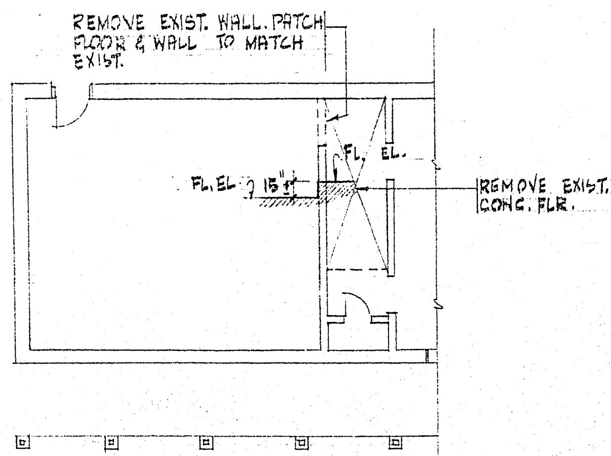
1 DEMOLITION PLAN Q-2 SCALE: 1/8" = 1'-0"
