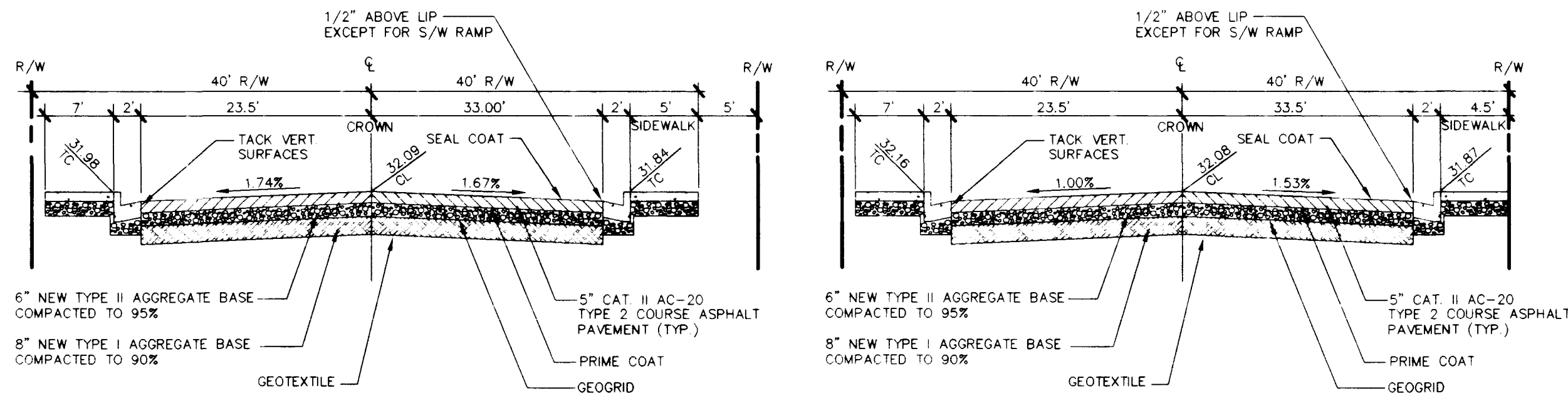
SECTION A-A STA. 9+00.00 N.T.S.
