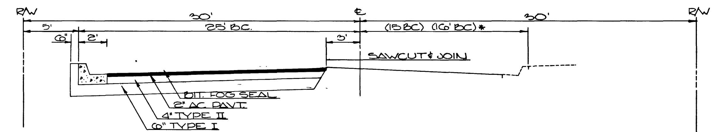
SECTION I 0+50-1+50 DESERT(N) 1+50-3+50
