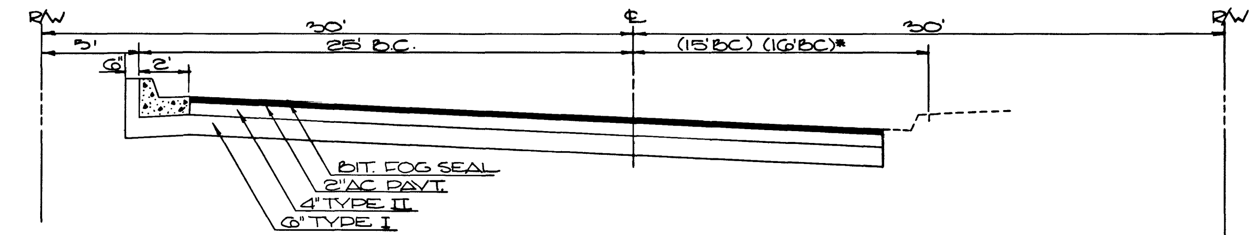
SECTION H 0+00-0+50 DESERT(N) 3+50-4+26.40
