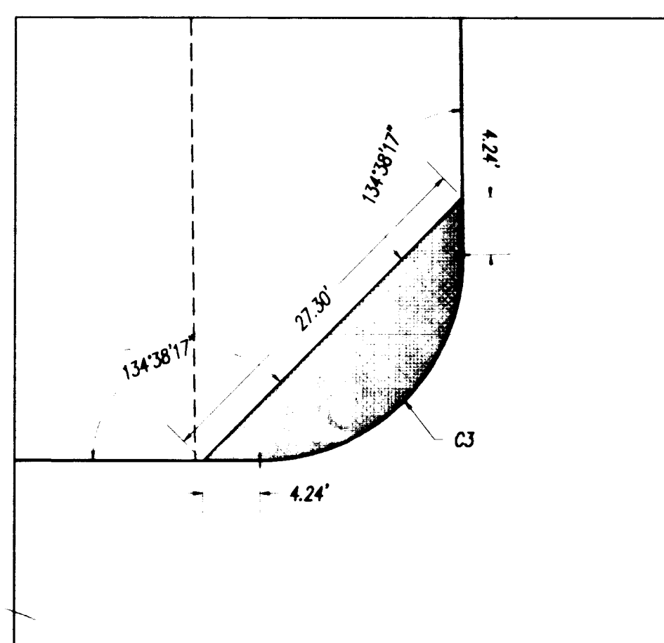
DETAIL 3 SCALE: 1"=10'
