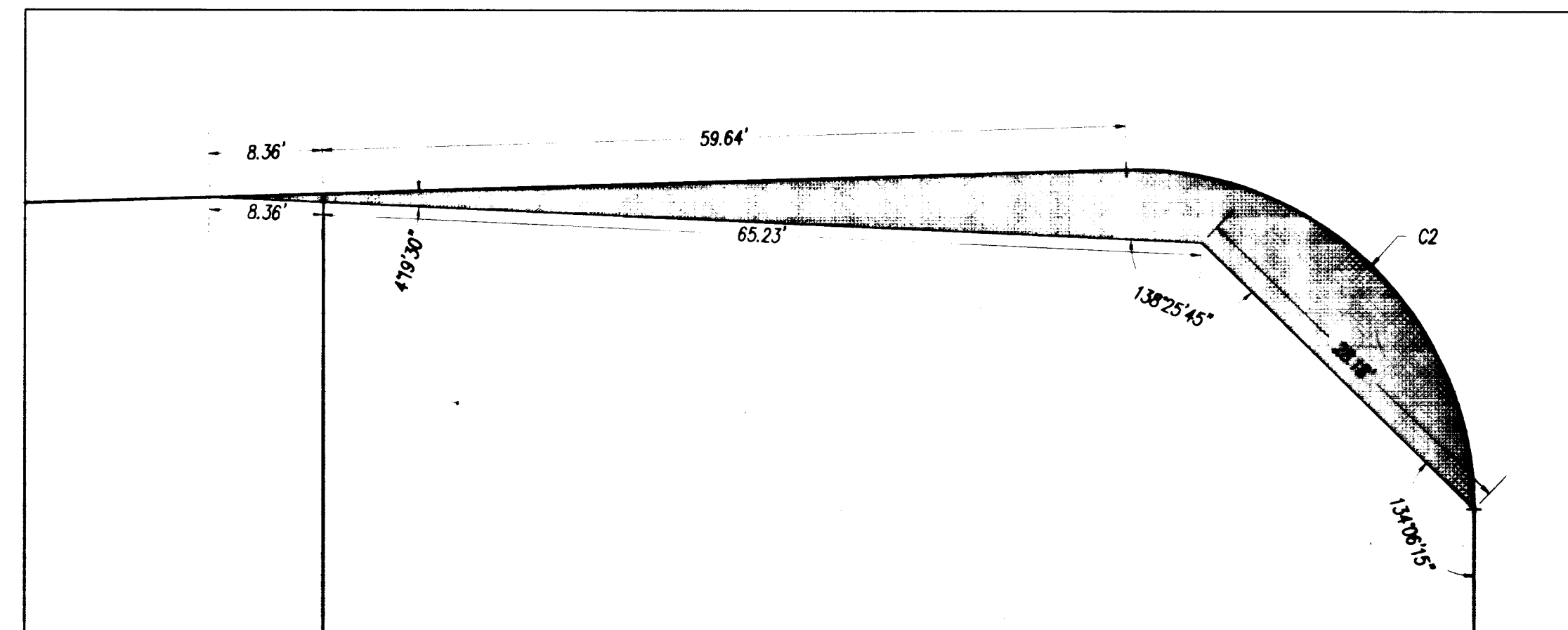
DETAIL 5 SCALE: 1"=10'
