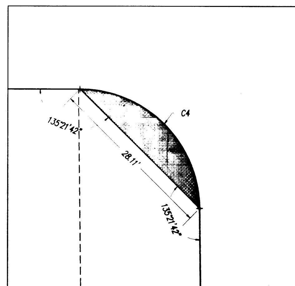
DETAIL 2 SCALE: 1"=10'
