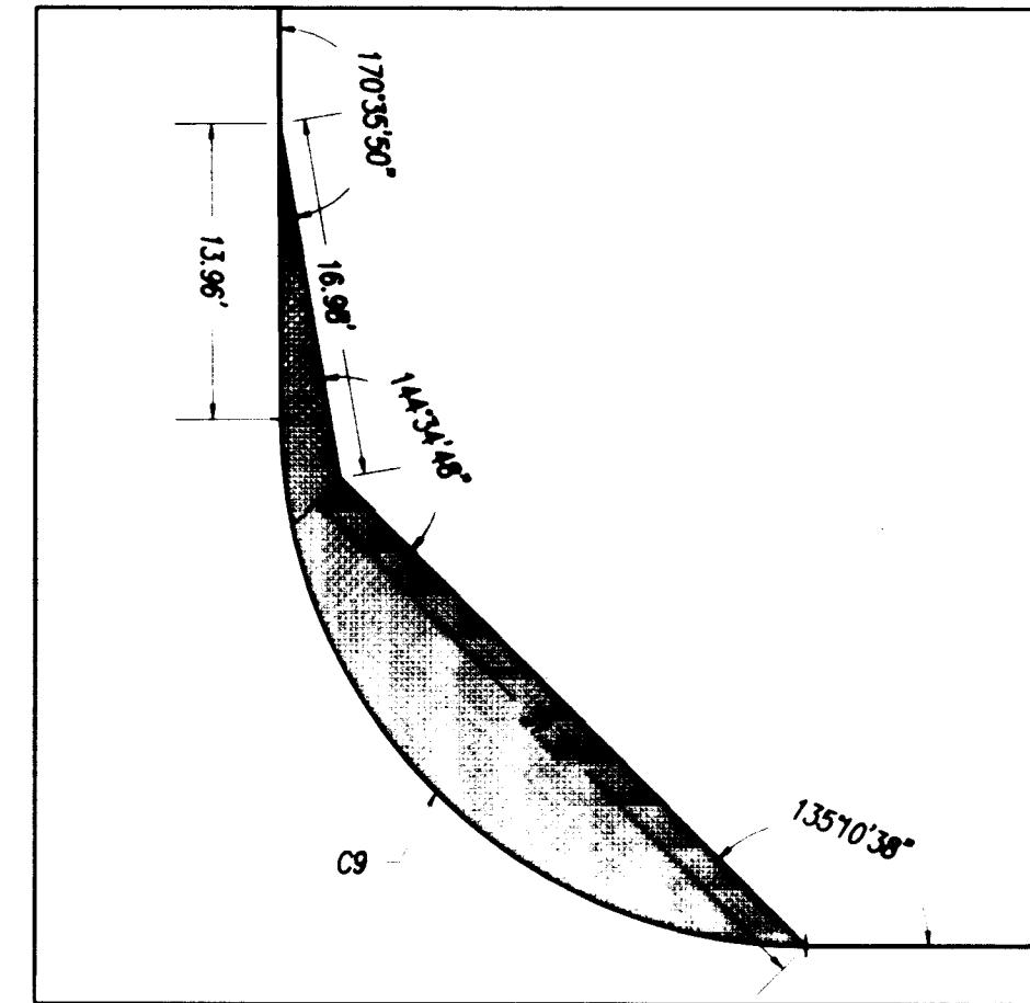
DETAIL 4 SCALE: 1"=10'
