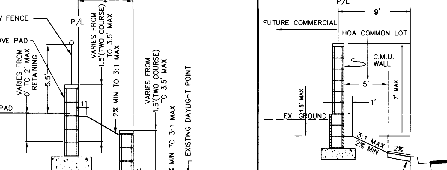
SECTION D1 - PASEO PARK
