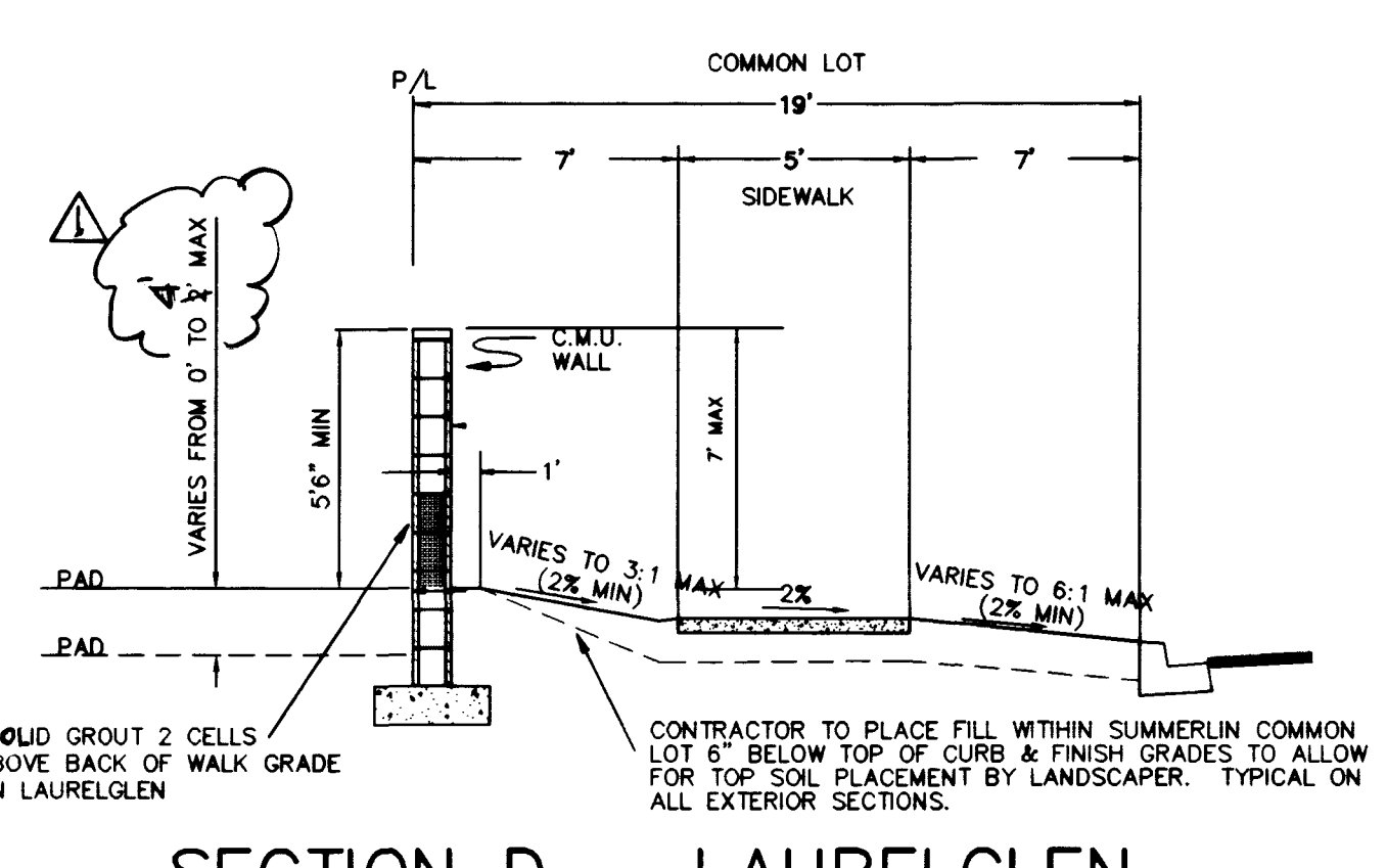
SECTION D - LAURELGLEN
