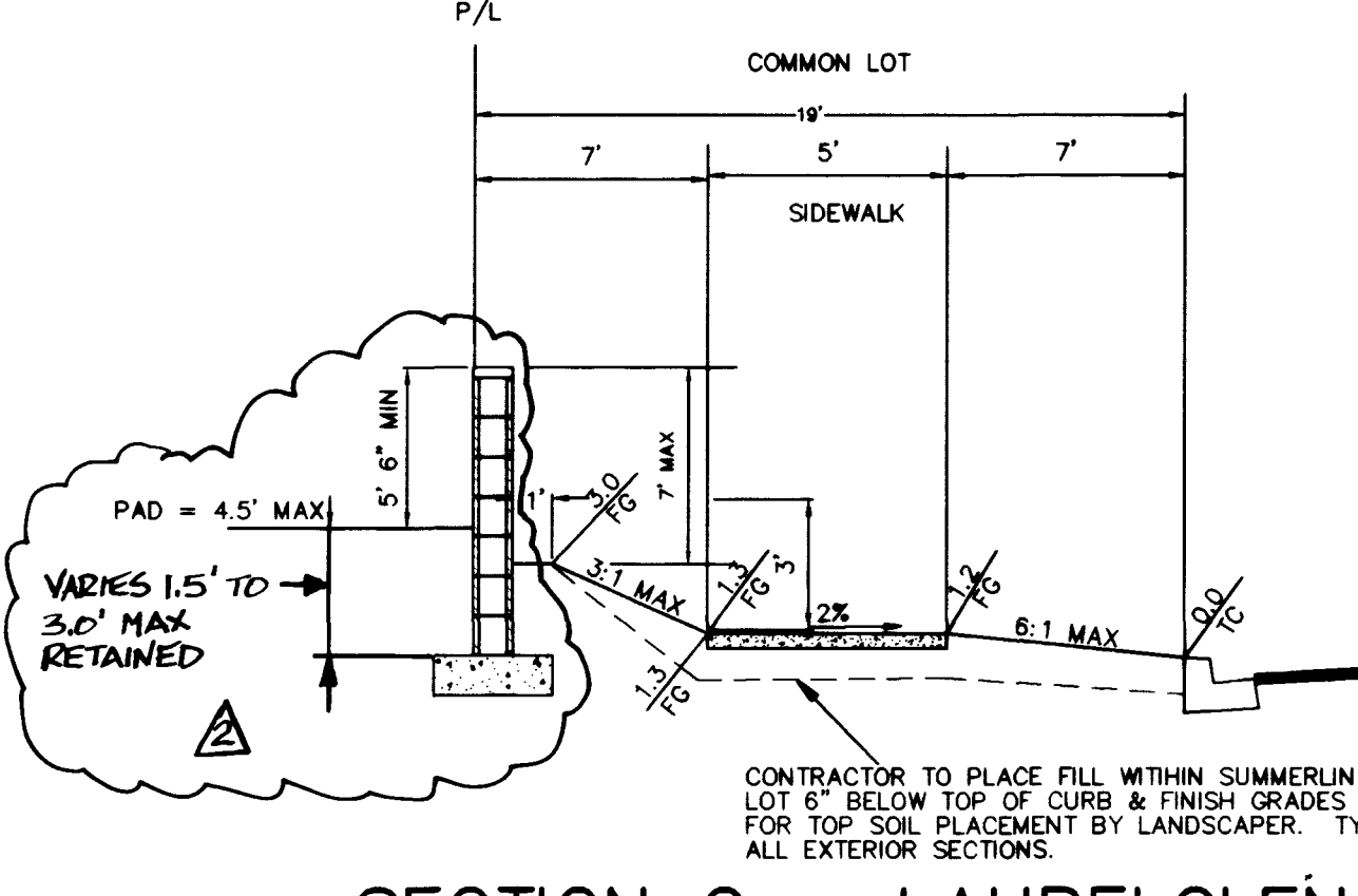
SECTION C - LAURELGLEN
