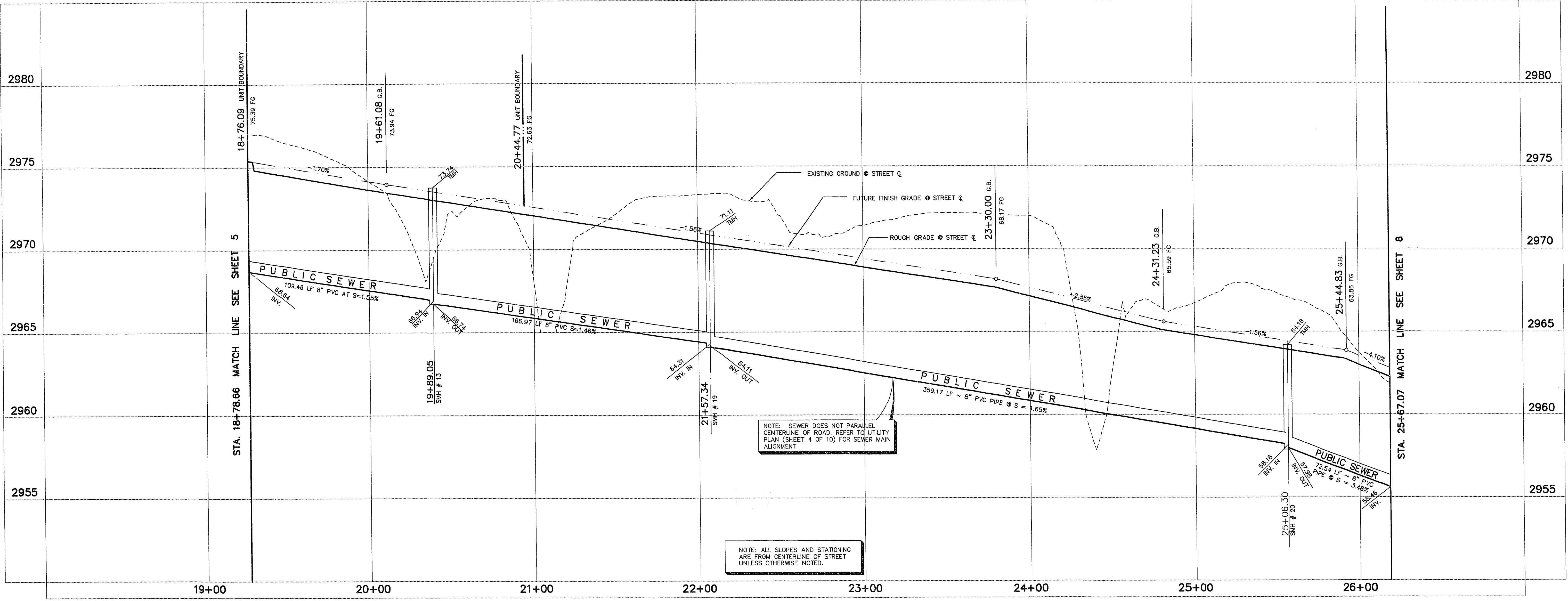
PROFILE HORIZ. 1" = 30' SCALE: VERT. 1" = 3'
