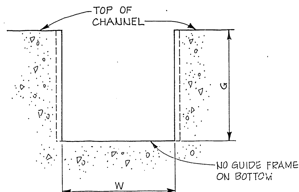
GUIDE ELEVATION (TYP)
