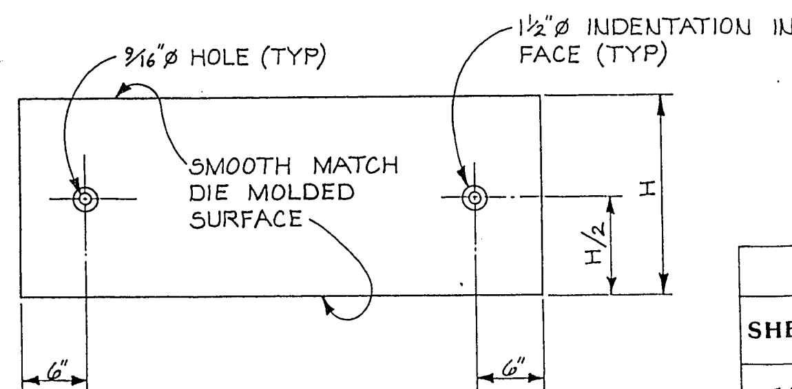
ELEVATION
