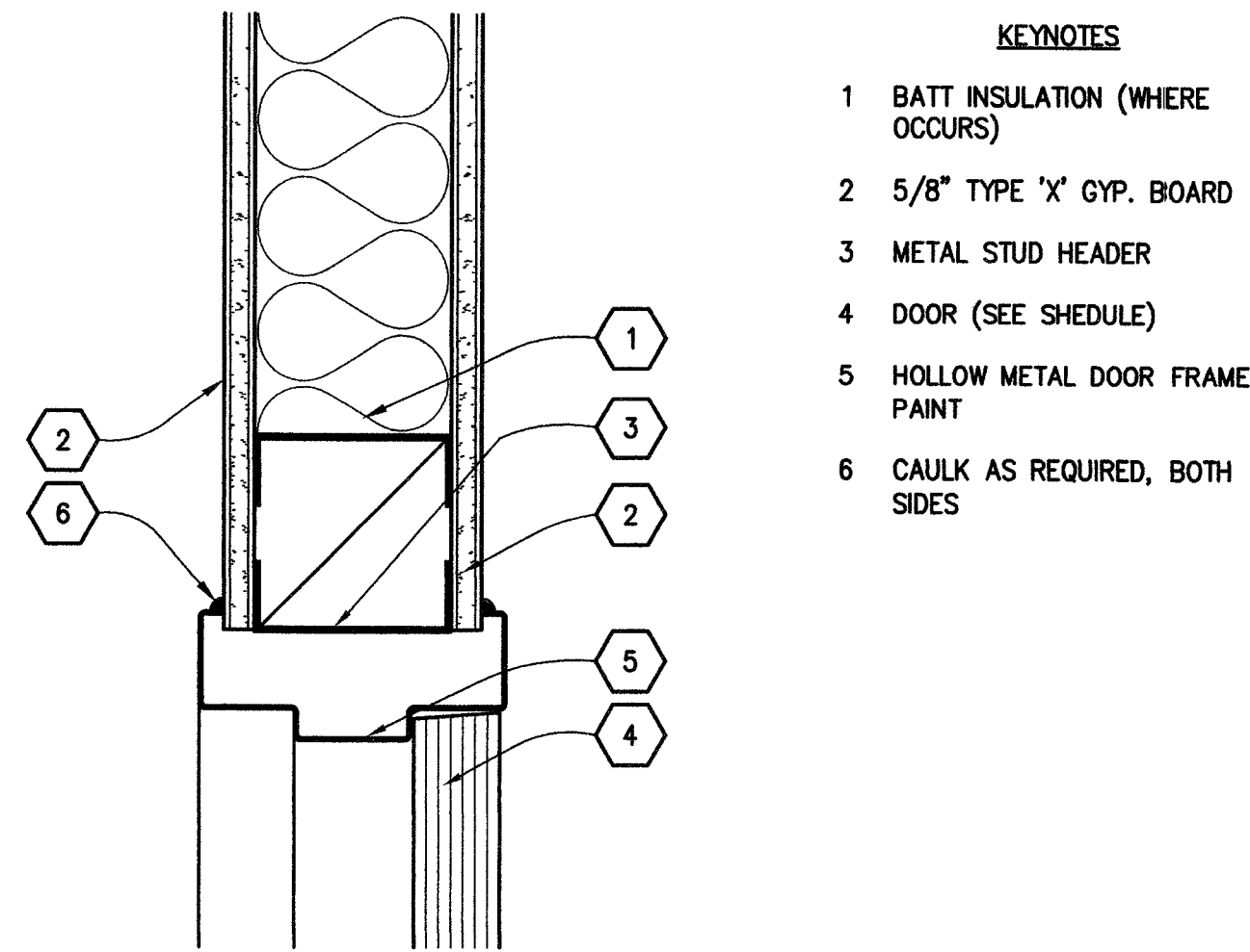
2 TYP. INTERIOR DOOR HEAD Scale: N.T.S. GA-9.3
