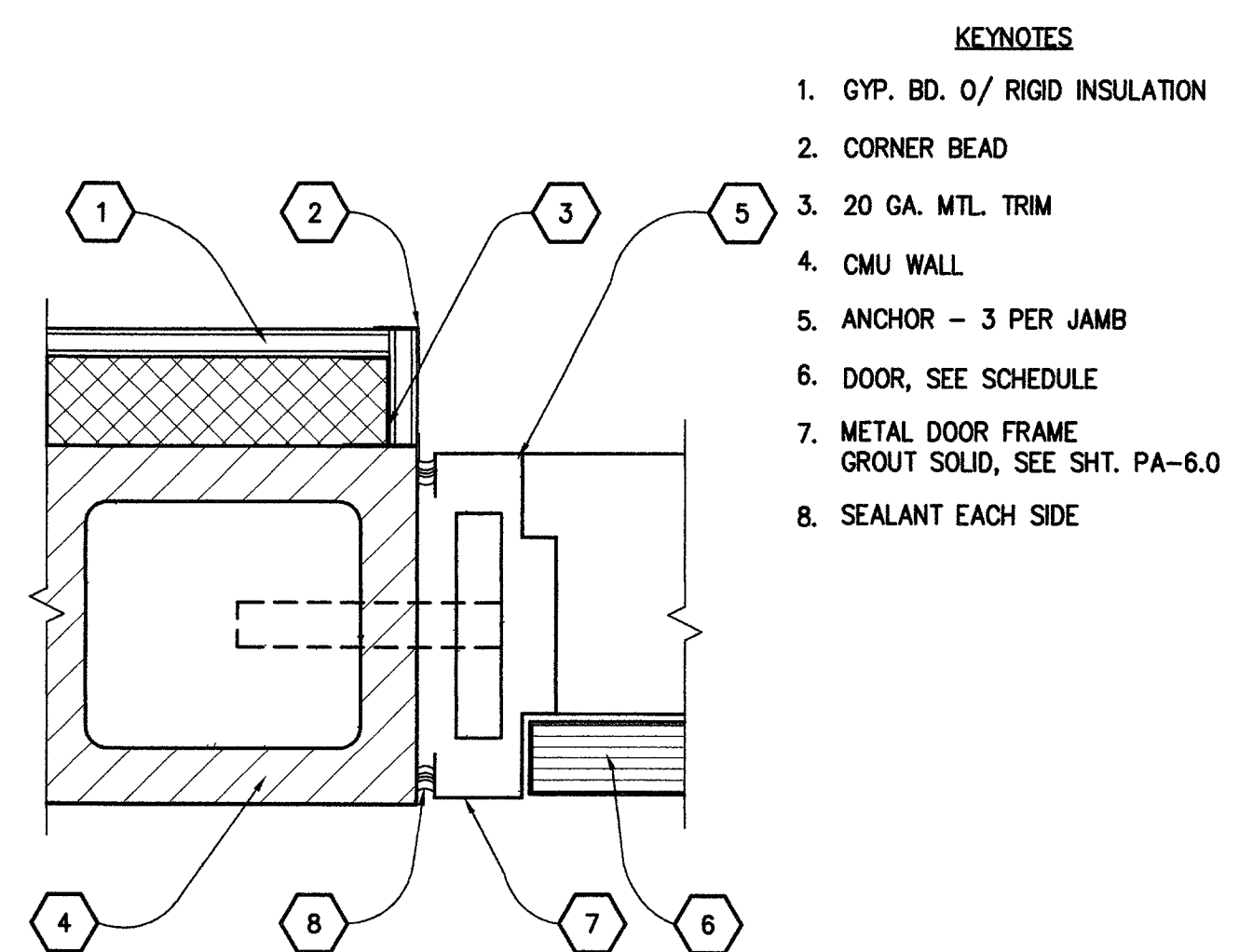
1 INTERIOR DOOR JAMB Scale: N.T.S. GA-9.3
