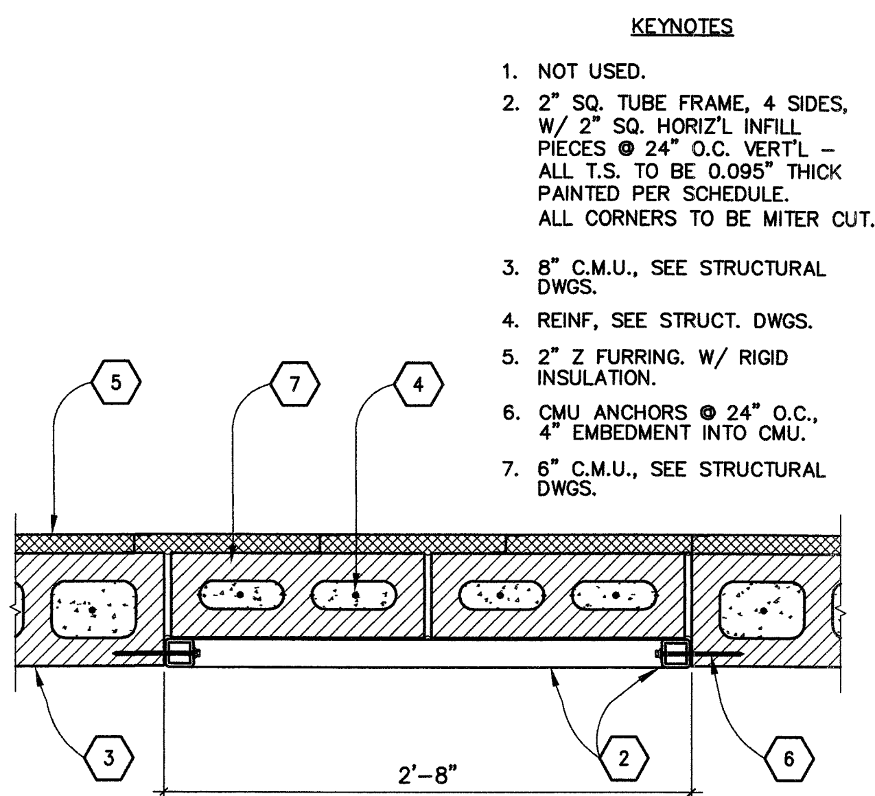
11 CMU NICHE DETAIL Scale: N.T.S.
