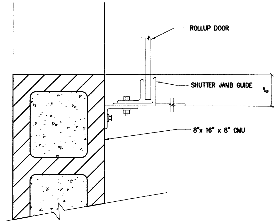
7 ROLL UP DOOR JAMB Scale: 3"=1'-0" GA-9.3
