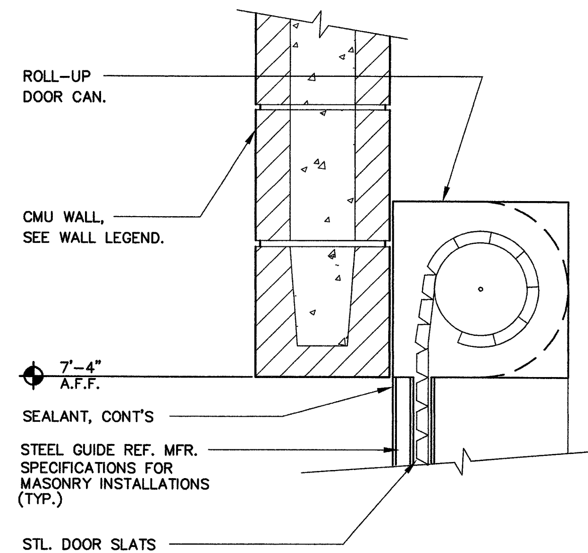
6 ROLL-UP DOOR HEAD Scale: N.T.S. GA-9.3
