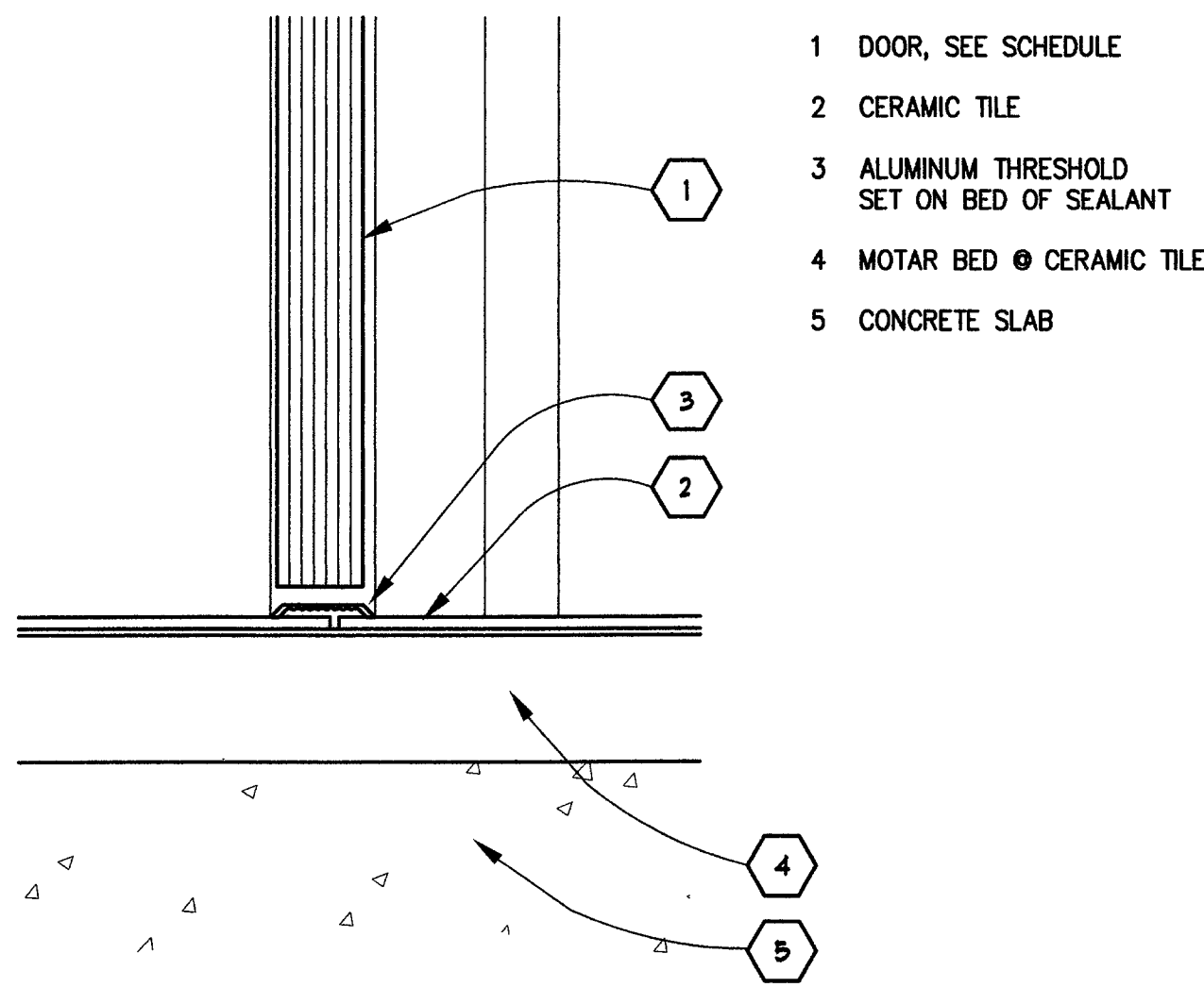
4 INTERIOR DOOR THRESHOLD Scale: N.T.S. GA-9.3
