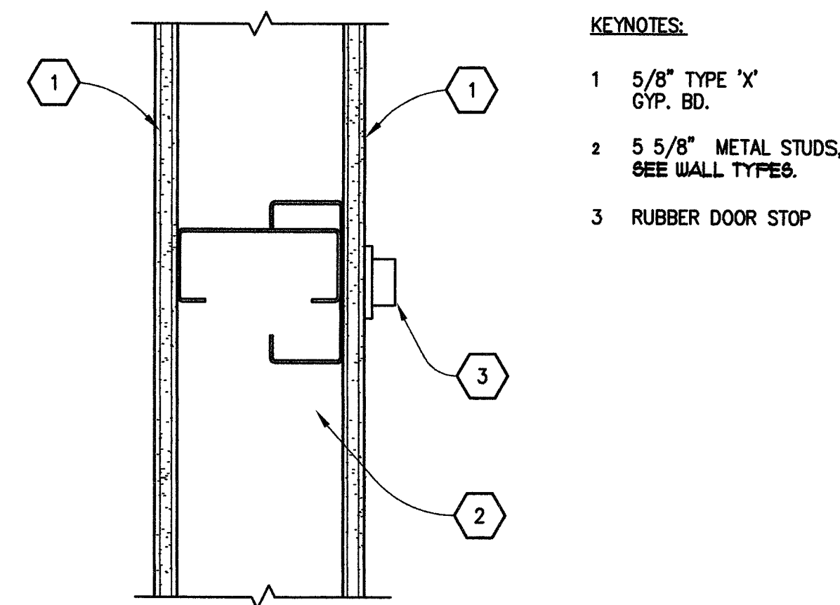
10 DOOR STOP Scale: N.T.S. GA-9.3
