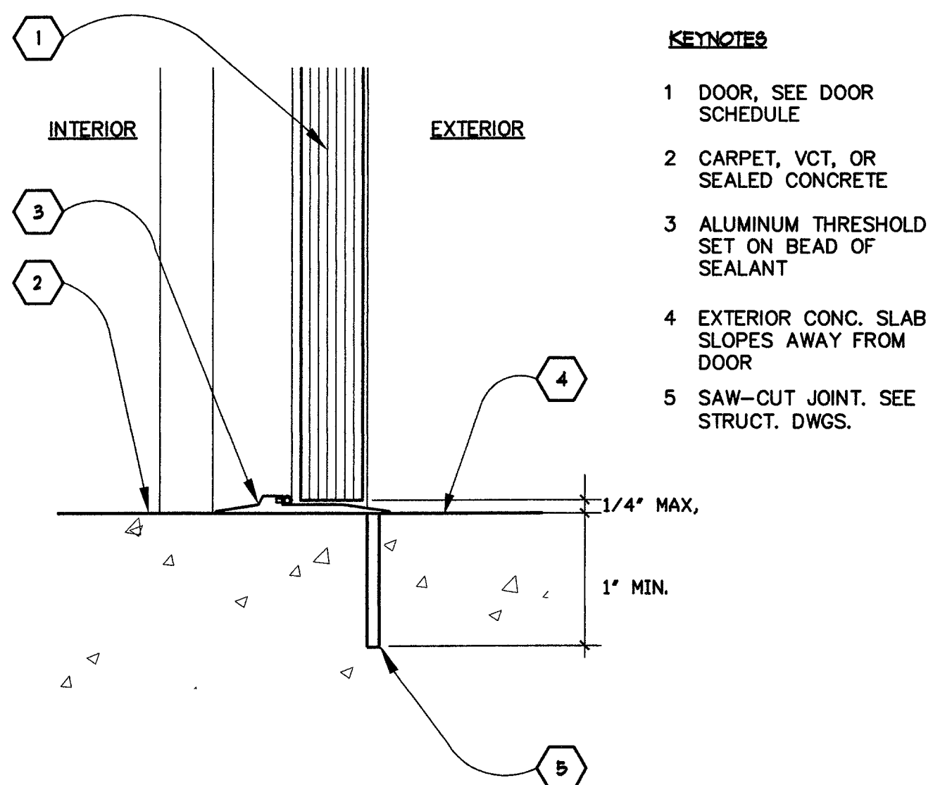
8 EXTERIOR DOOR SILL Scale: N.T.S. GA-9.3
