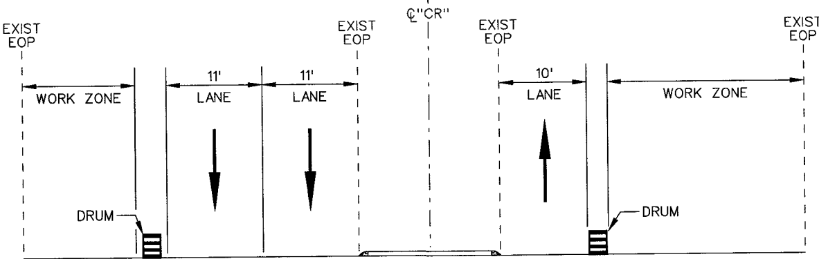
SECTION D-O
