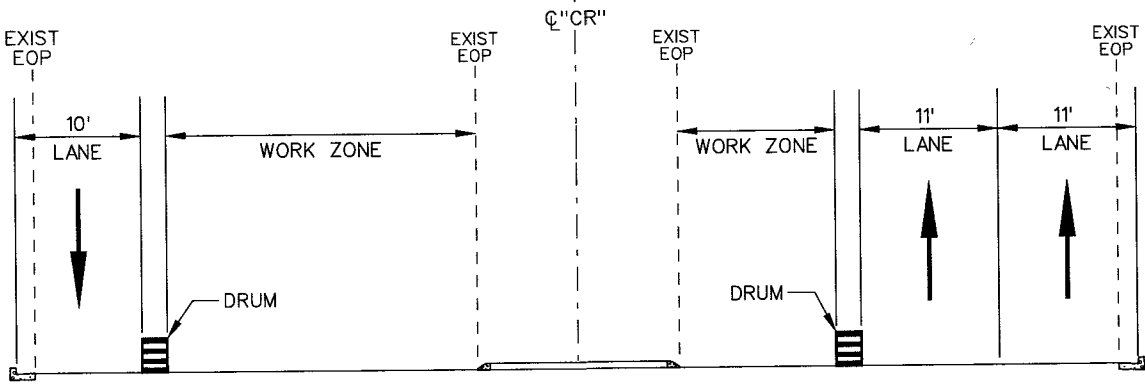
SECTION D-Q
