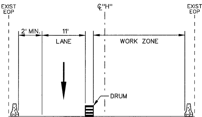
SECTION C-V
