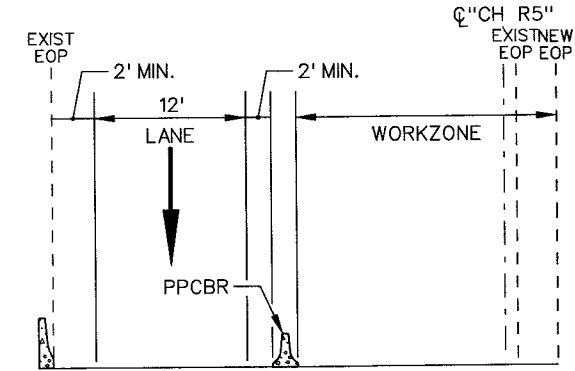
SECTION D-V
