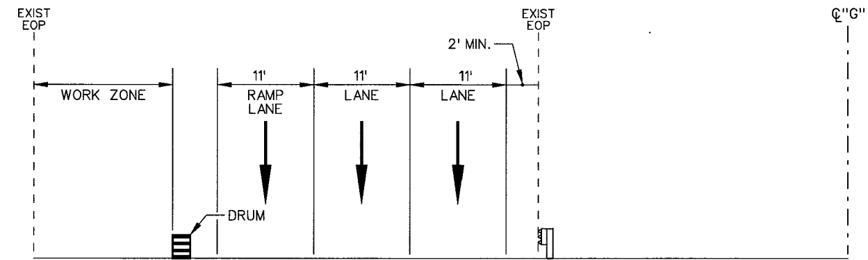
SECTION D-D
