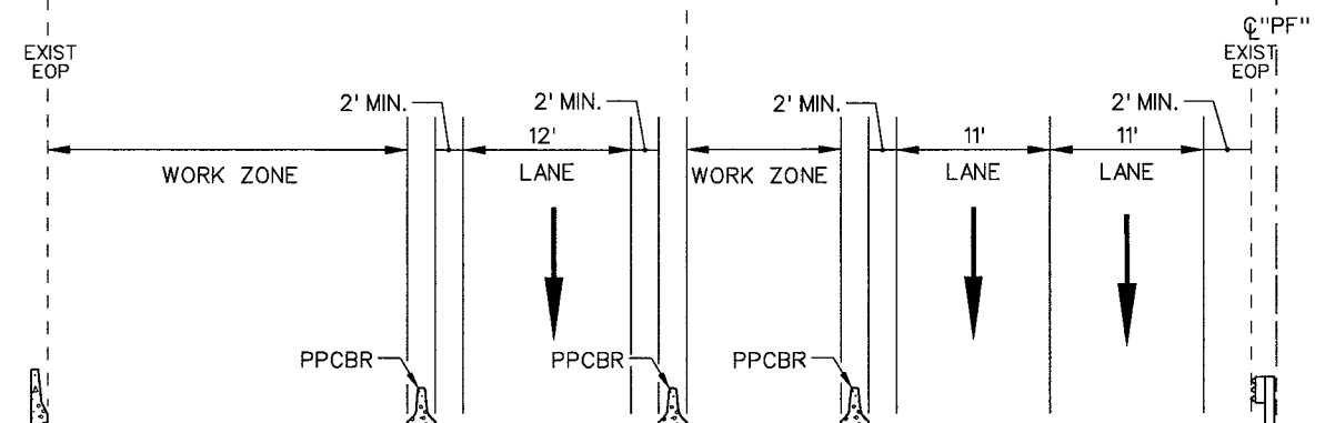
SECTION D-M2
