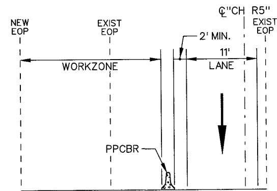
SECTION D-S
