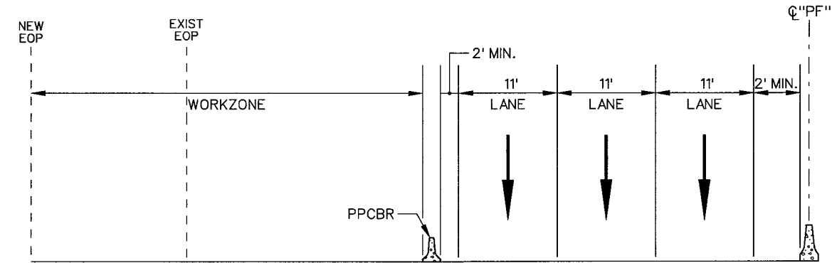
SECTION E-I
