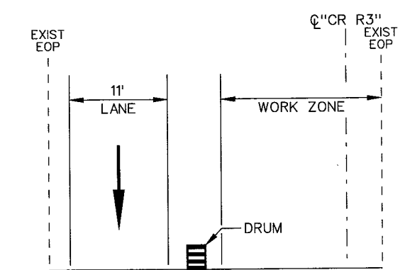
SECTION D-I
