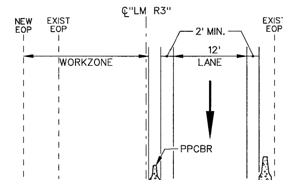
SECTION E-J
