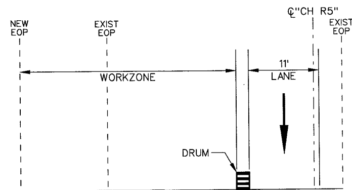
SECTION D-T
