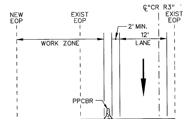
SECTION D-E
