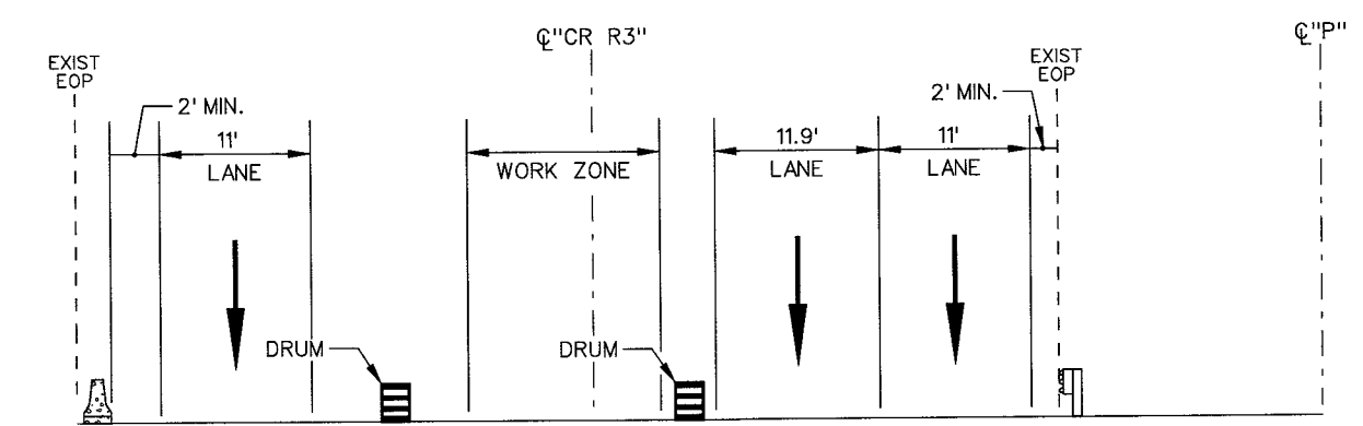
SECTION D-J
