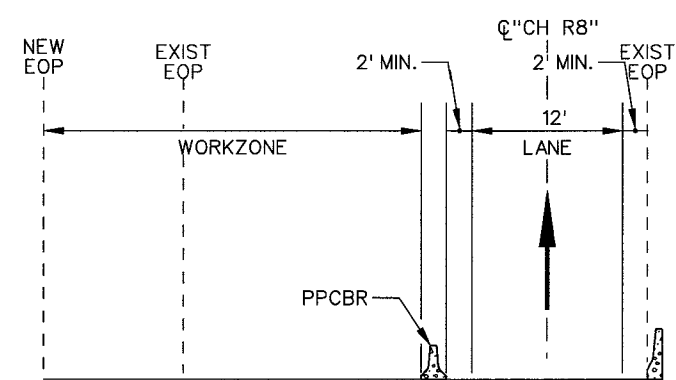
SECTION B-I
