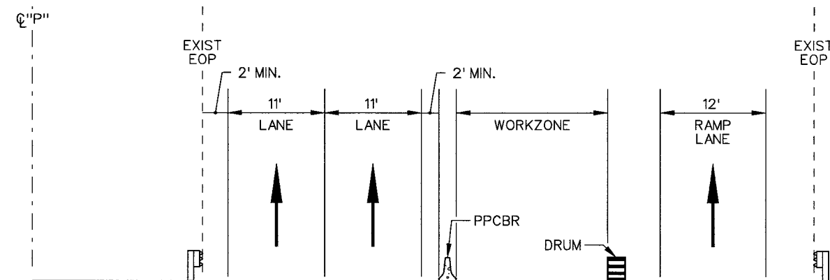
SECTION C-D
