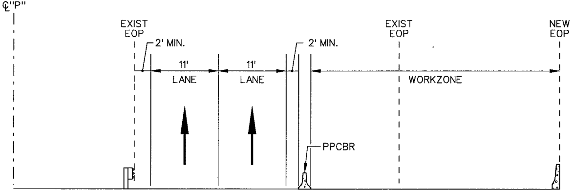
SECTION C-A
