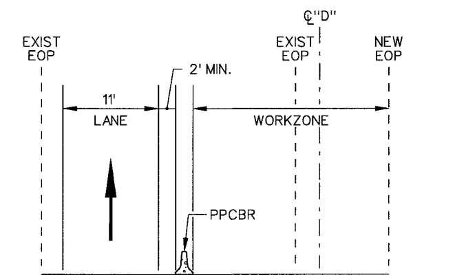
SECTION C-E
