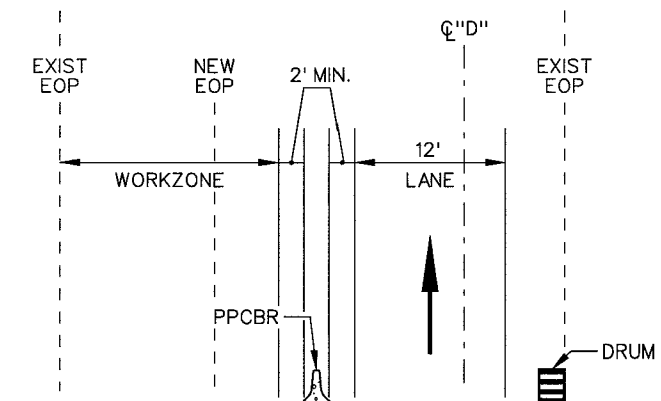
SECTION C-F
