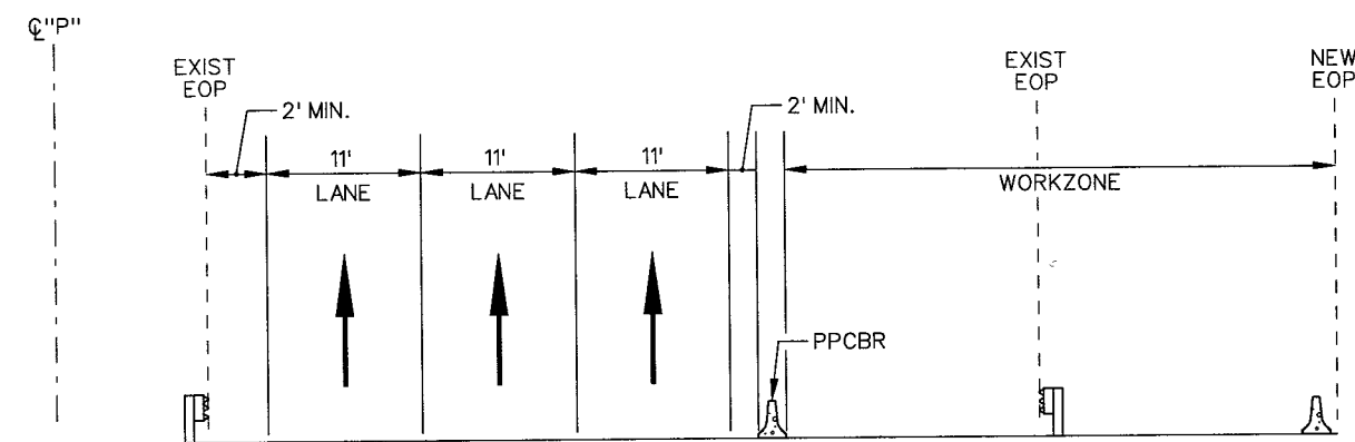
SECTION C-I
