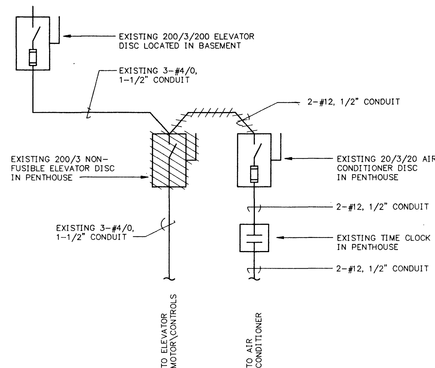
ELEVATOR EXISTING ONE LINE DIAGRAM SCALE: N.T.S.
