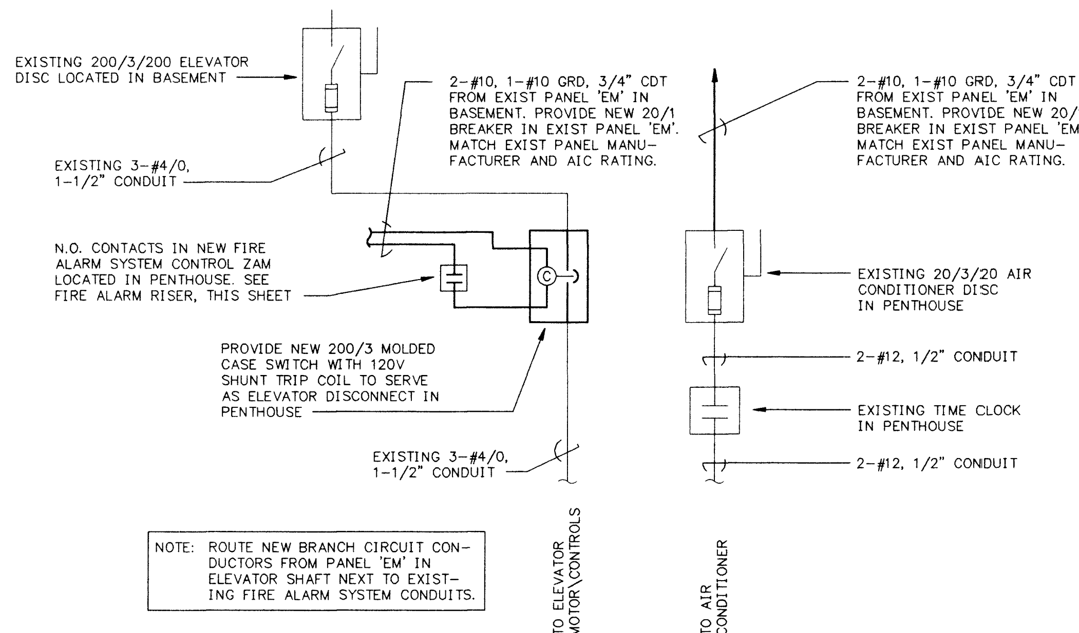
ELEVATOR EXISTING ONE LINE DIAGRAM SCALE: N.T.S.
