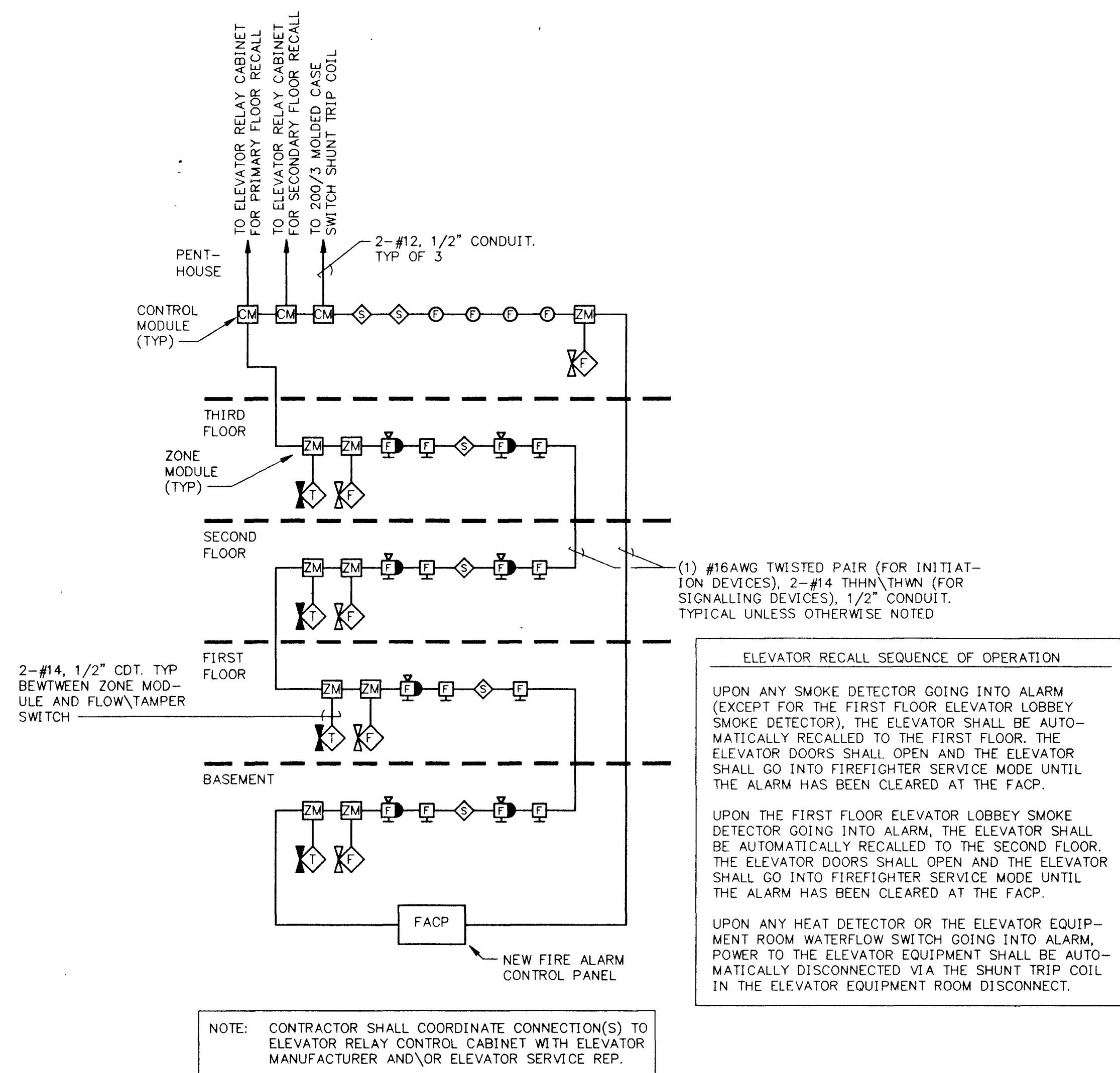
ELEVATOR EXISTING ONE LINE DIAGRAM SCALE: N.T.S.
