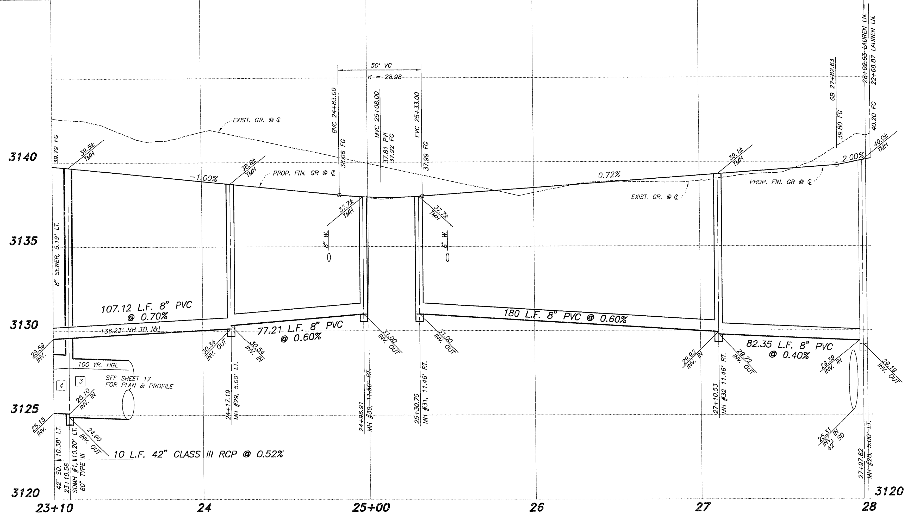
PROFILE SCALE: HORIZ. 1" = 30' VERT. 1" = 3'
