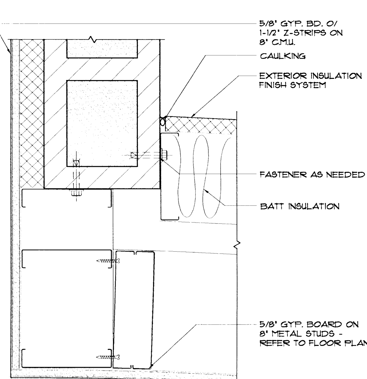
WALL INTERSECTION SCALE: 3" = 1'-0"
