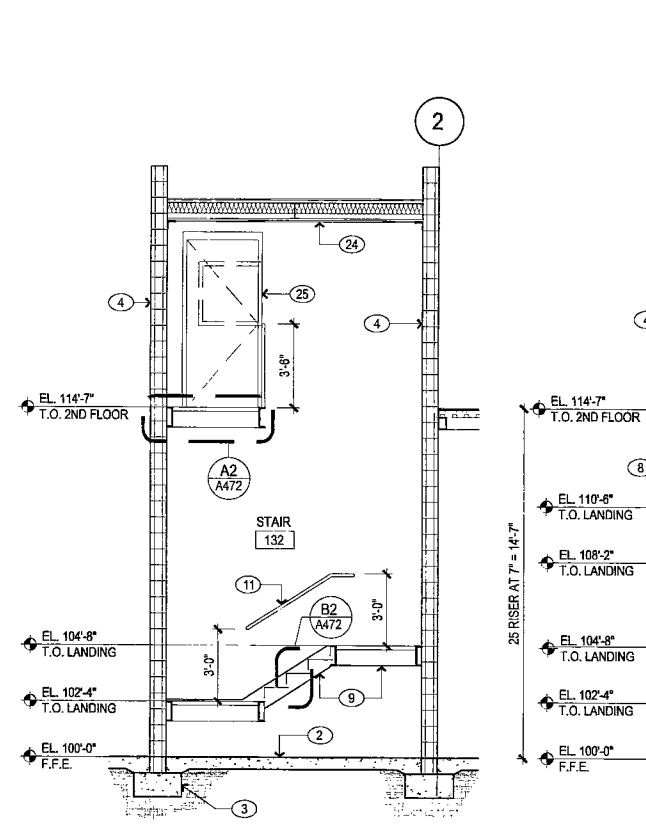
E3 STAIR SECTION
