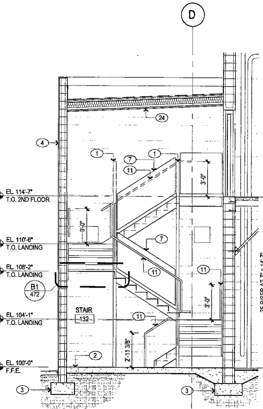
E1 STAIR SECTION
