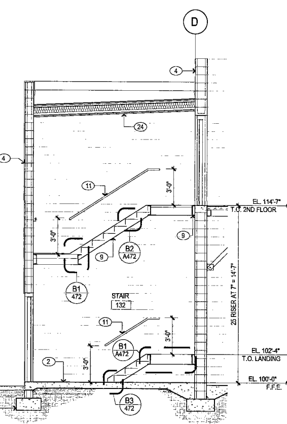
E2 STAIR SECTION
