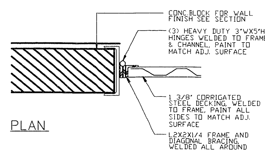
K TRASH ENCLOSURE DOOR NO SCALE
