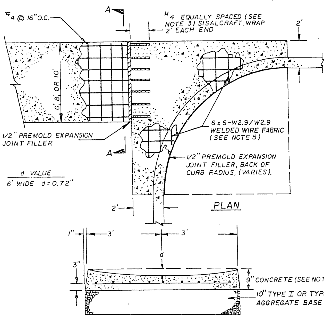
SECTION A-A
