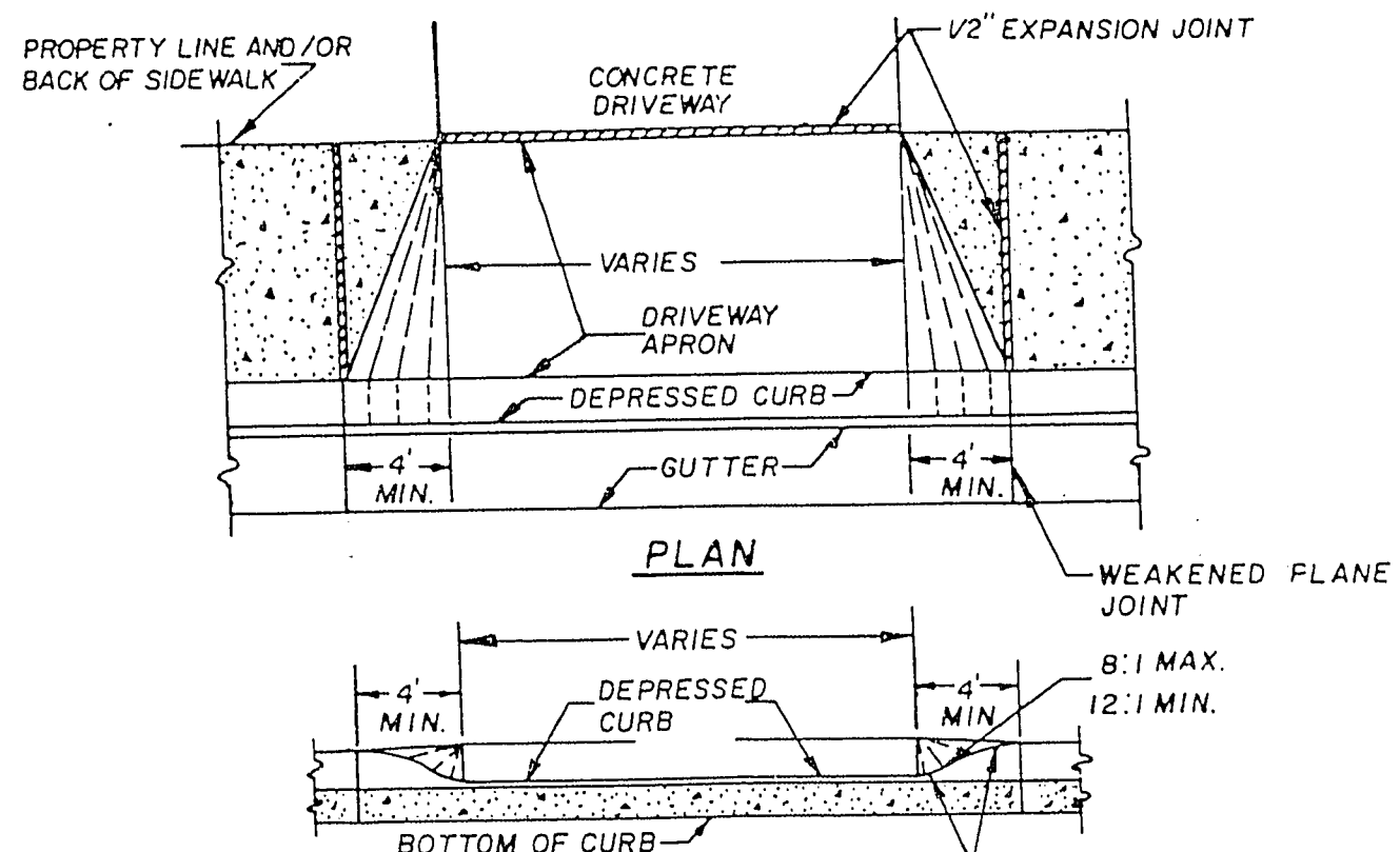
ELEVATION
