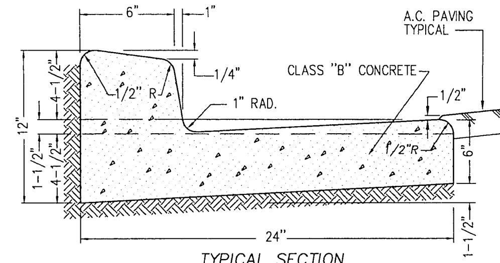
G "L" TYPE CURB AND GUTTER N.T.S.
