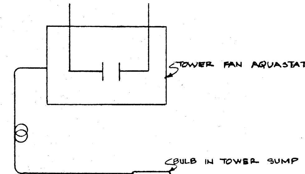
TOWER FAN CONTROL NO SCALE
