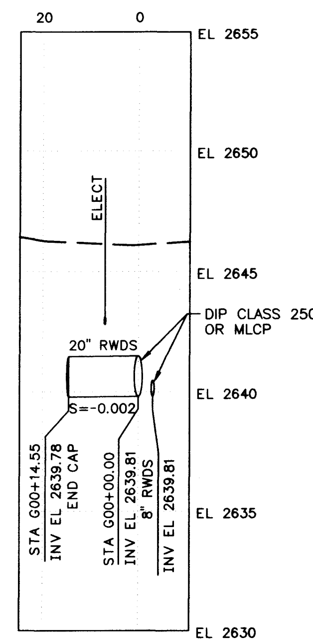
TURNOUT 'G' - 20" AT STA 140+10.81 (7) (C12)
