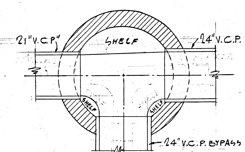
PLAN M.H. @ 33+60 (BYPASS M.H. SIMILAR)
