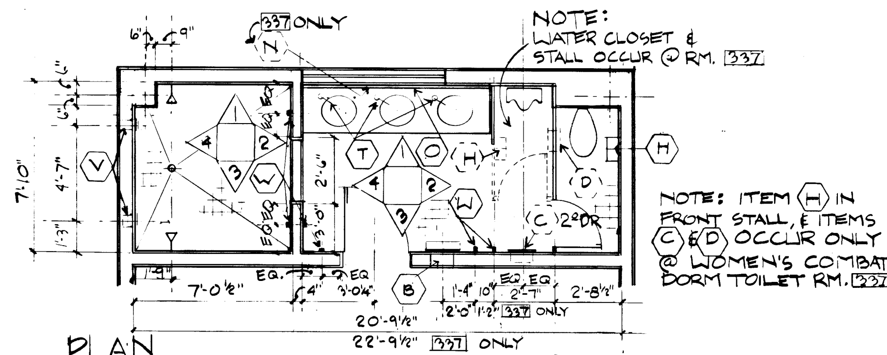
PLAN 1/4"=1'-0"
