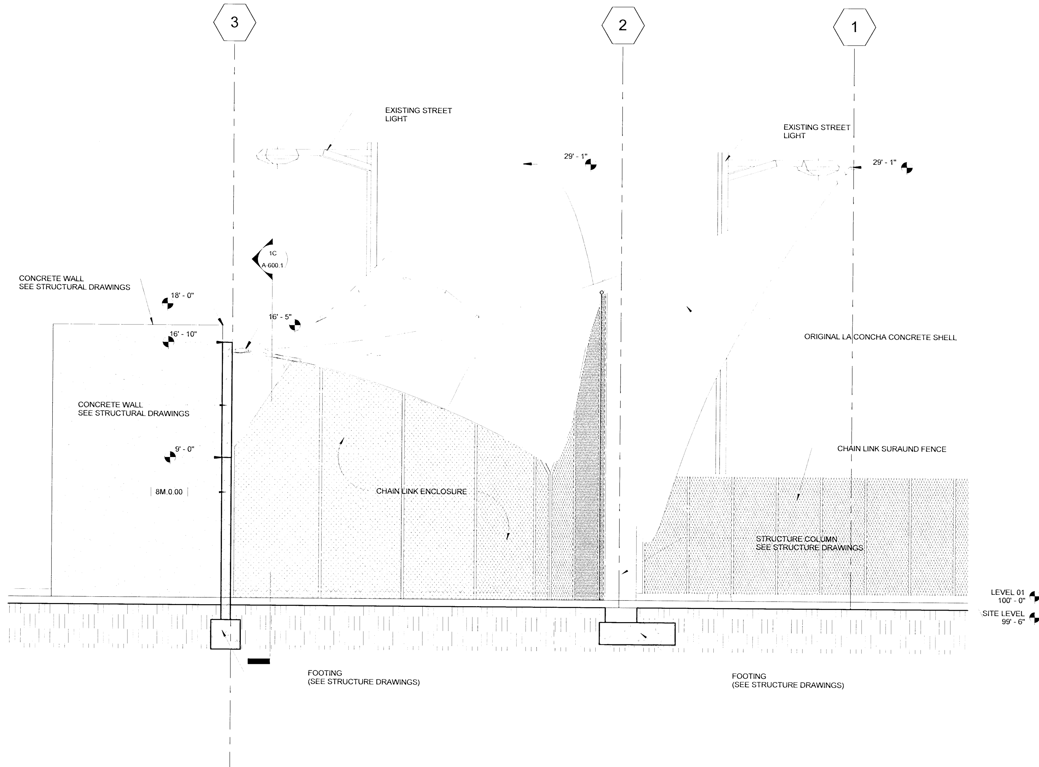
1E OVERALL LONGITUDE SECTION
