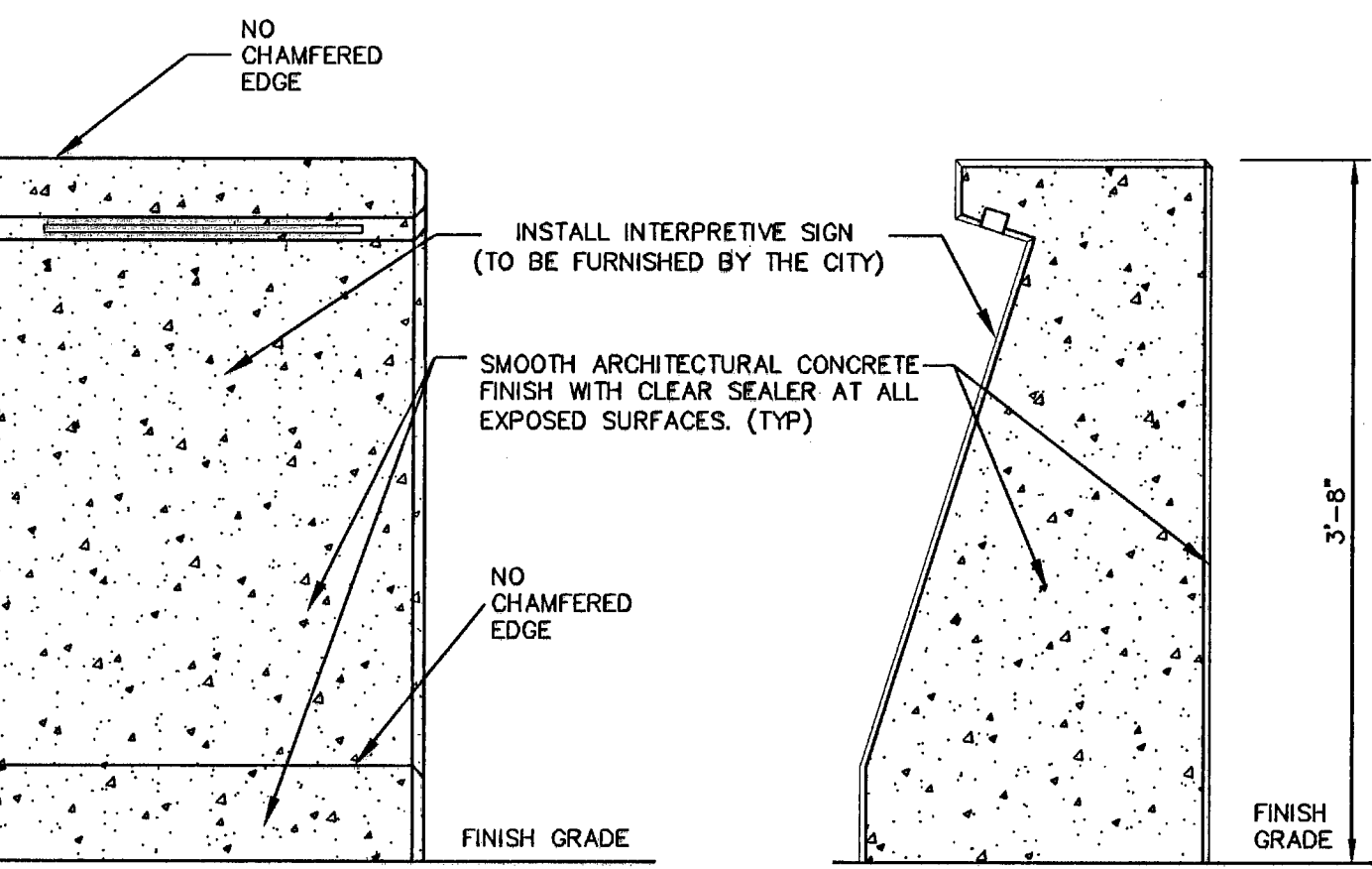
SECTION - CONCRETE MONUMENT FOR INTERPRETIVE SIGN N.T.S.
