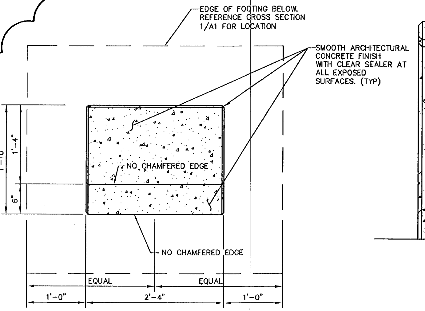
TOP VIEW - CONCRETE MONUMENT FOR INTERPRETIVE SIGN N.T.S.
