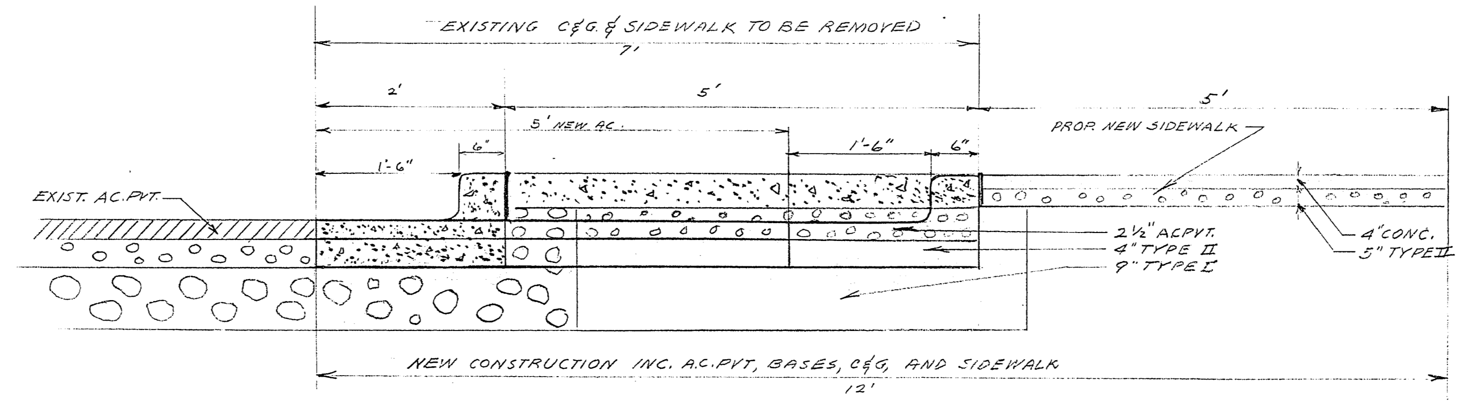
SEC. A-A
