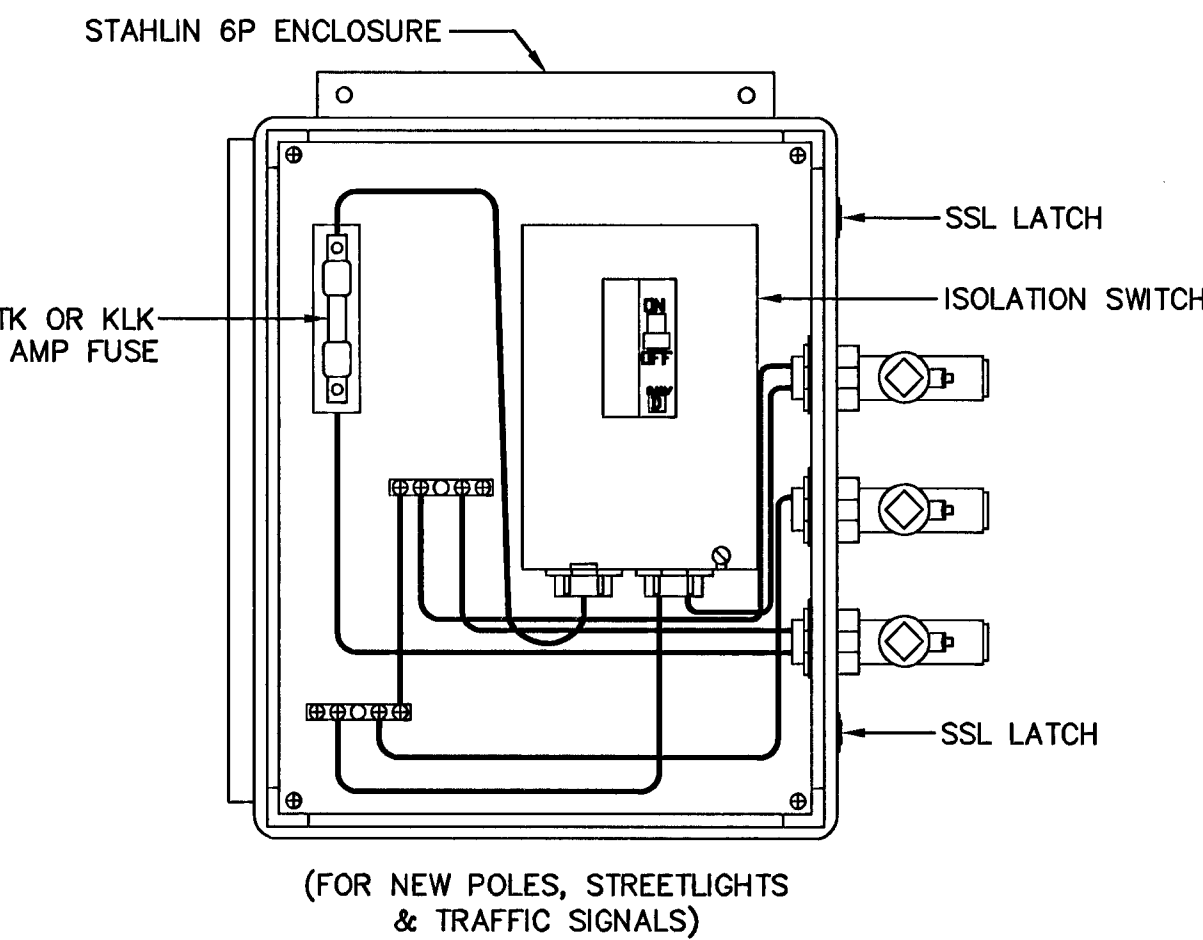
WTR FUSE BOX NTS
