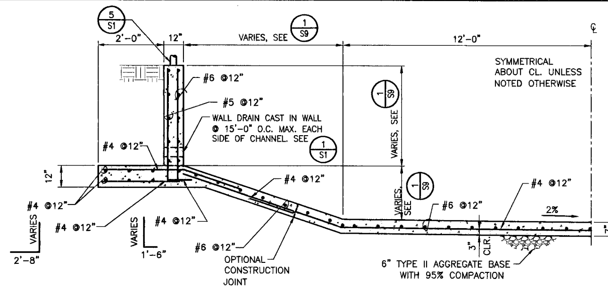
WALL SECTION A SCALE: 1/2"=1'-0"
