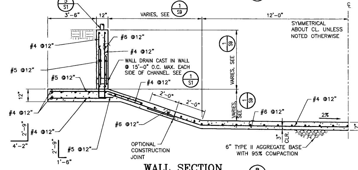
WALL SECTION B SCALE: 1/2"=1'-0"
