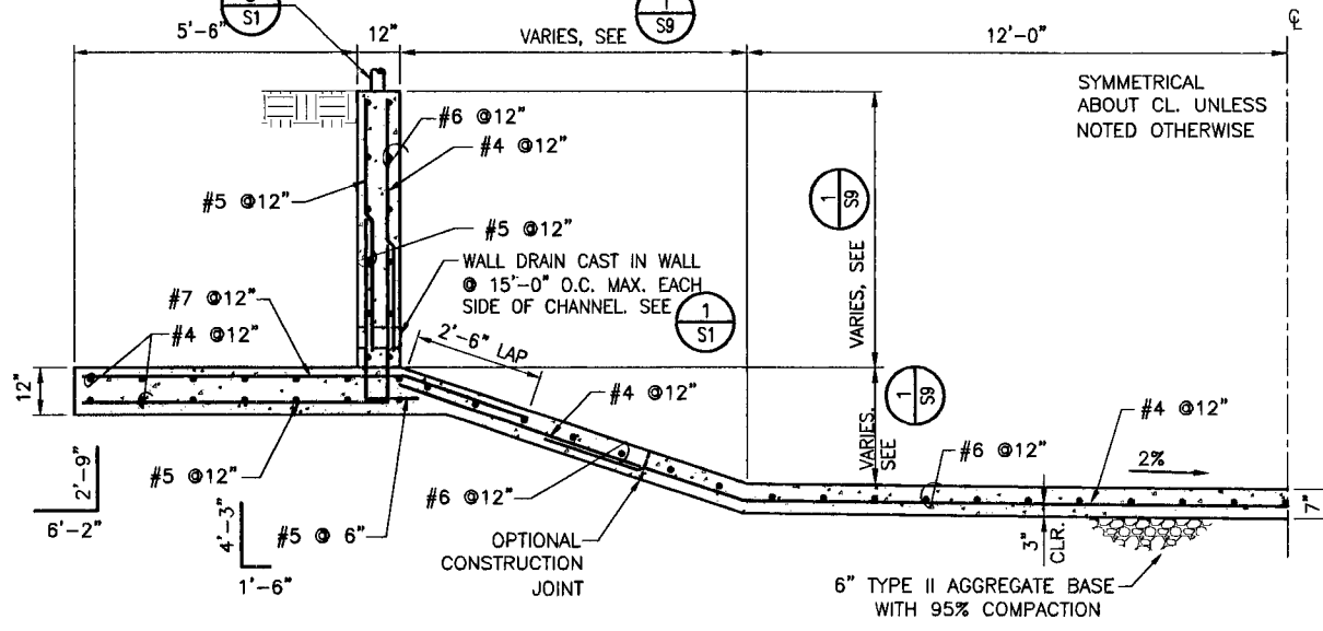
WALL SECTION C SCALE: 1/2"=1'-0"
