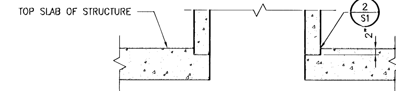
MANHOLE RISER DETAIL
