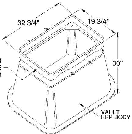
SCALE: N.T.S. 17" X 30" CONNECTOR VAULT
