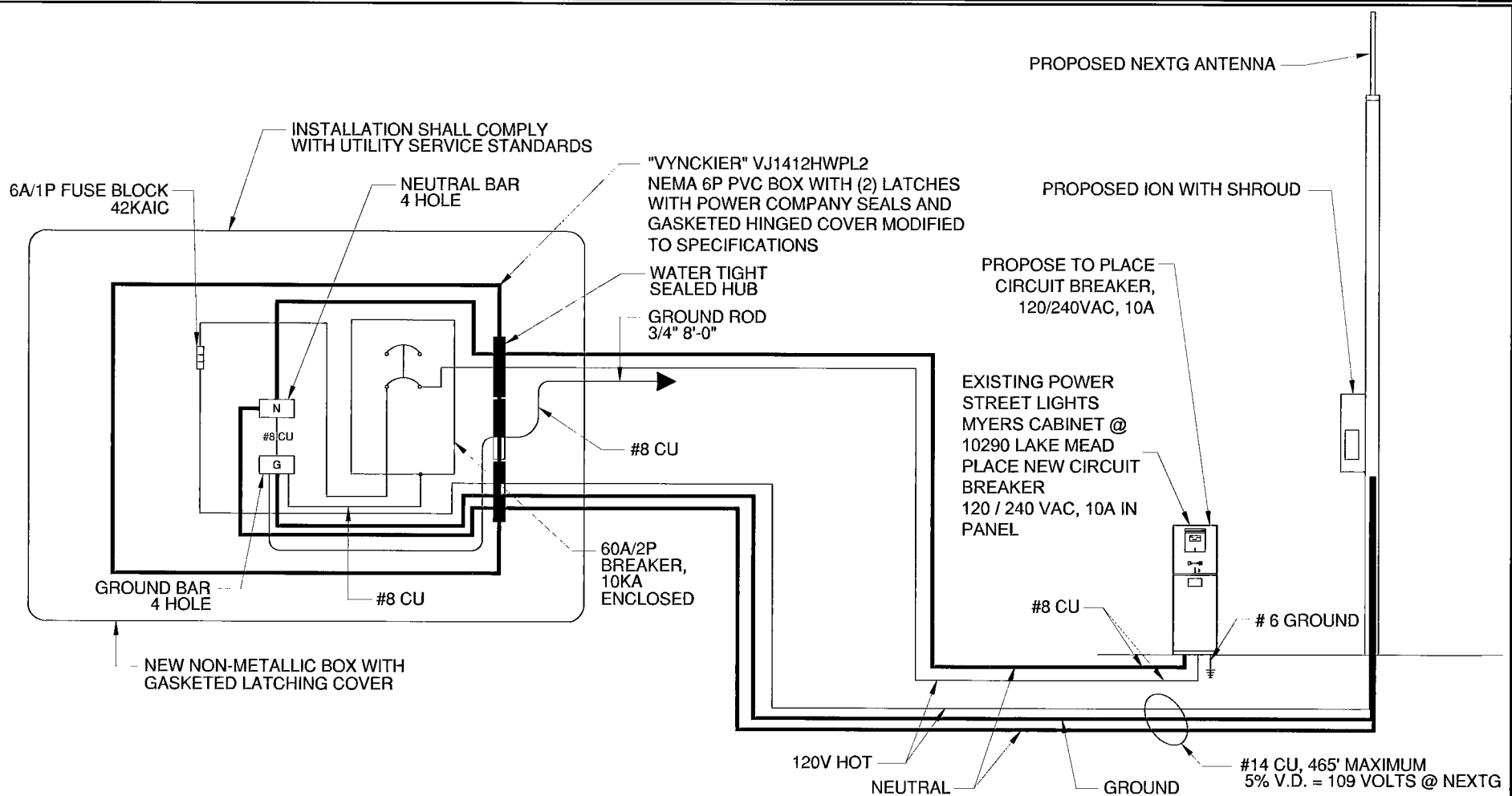
SCALE: N.T.S. POWER SINGLE LINE DIAGRAM
