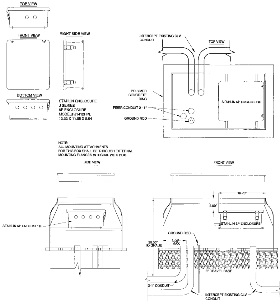
SCALE: N.T.S. STAHLIN 6P ENCLOSURE
