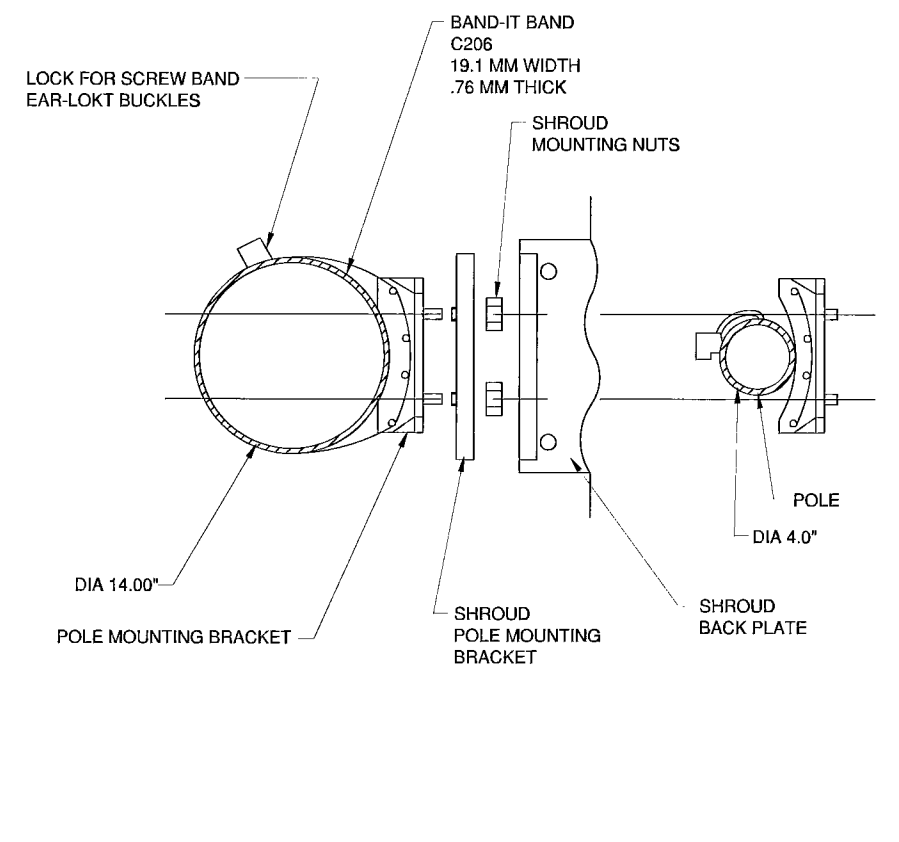
SCALE: N.T.S. POLE MOUNTING PER AMERON STANDARDS
