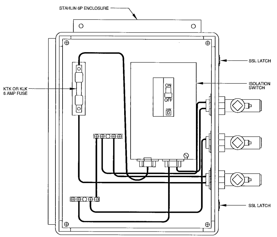
122722 SCALE: N.T.S. POWER SERVICE DISCONNECT FUSE BOX
