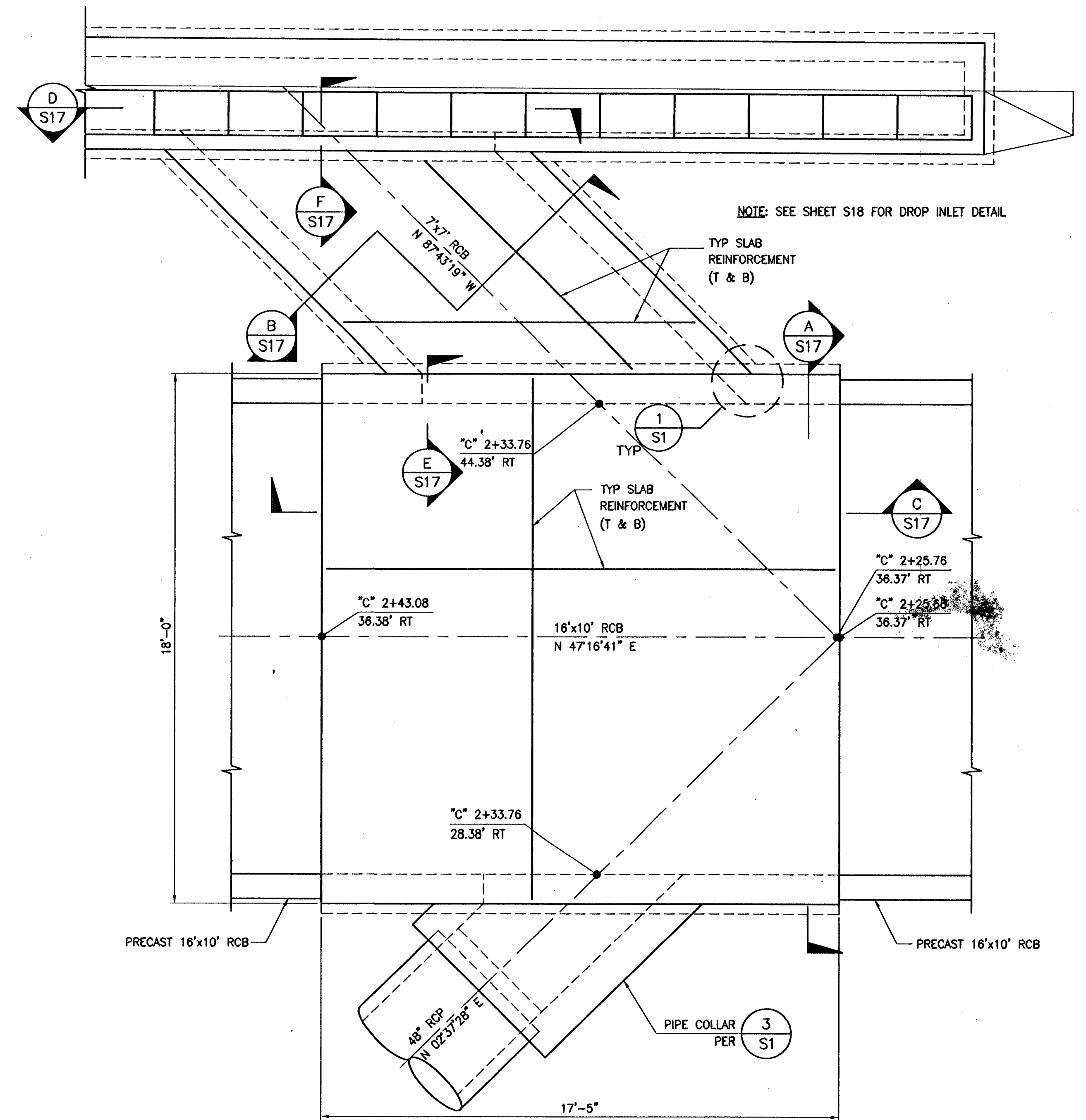
1 PLAN SCALE: 3/8" = 1'-0"
