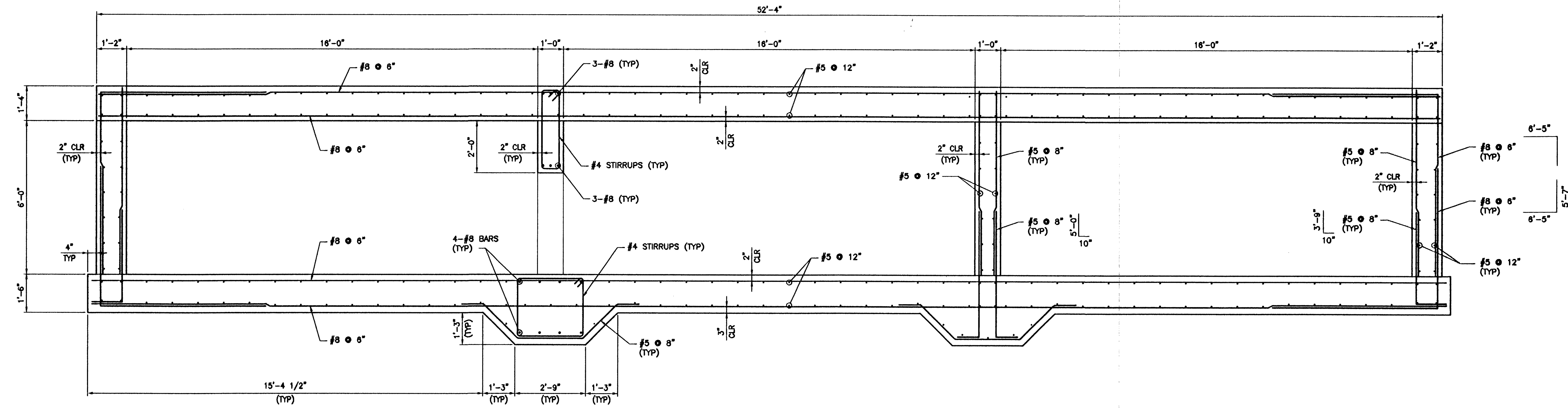
A SECTION SCALE: 1/2" = 1'-0"
