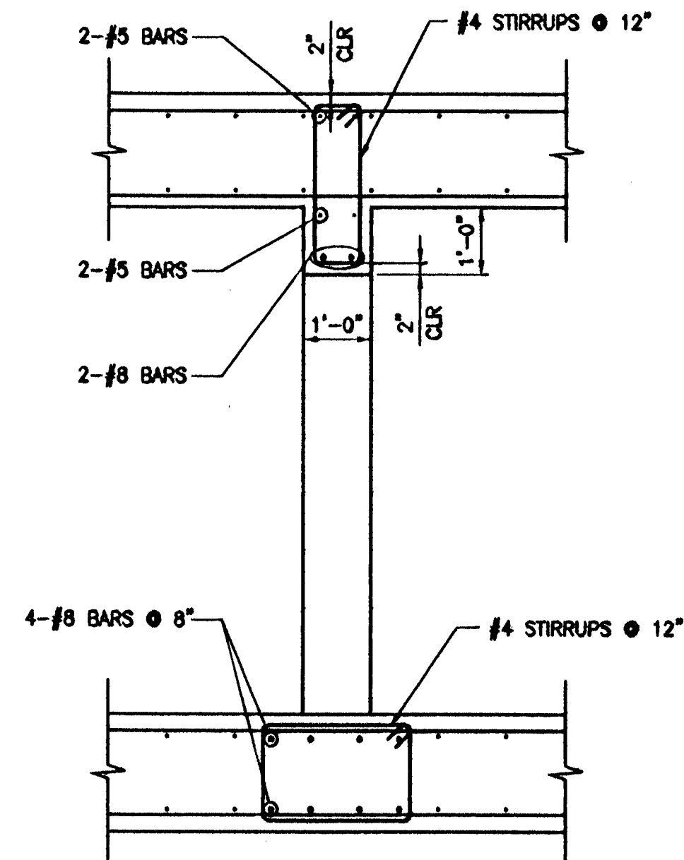
B SECTION SCALE: 1/2" = 1'-0"
