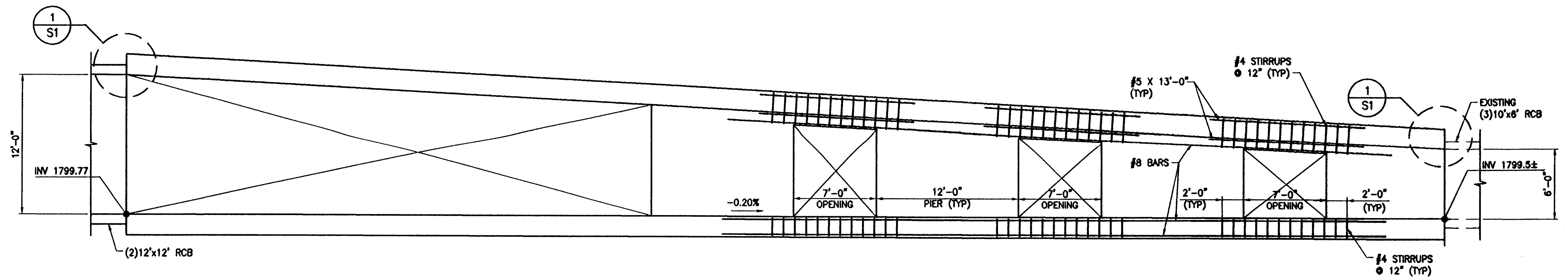
A SECTION SCALE: 3/16" = 1'-0"
