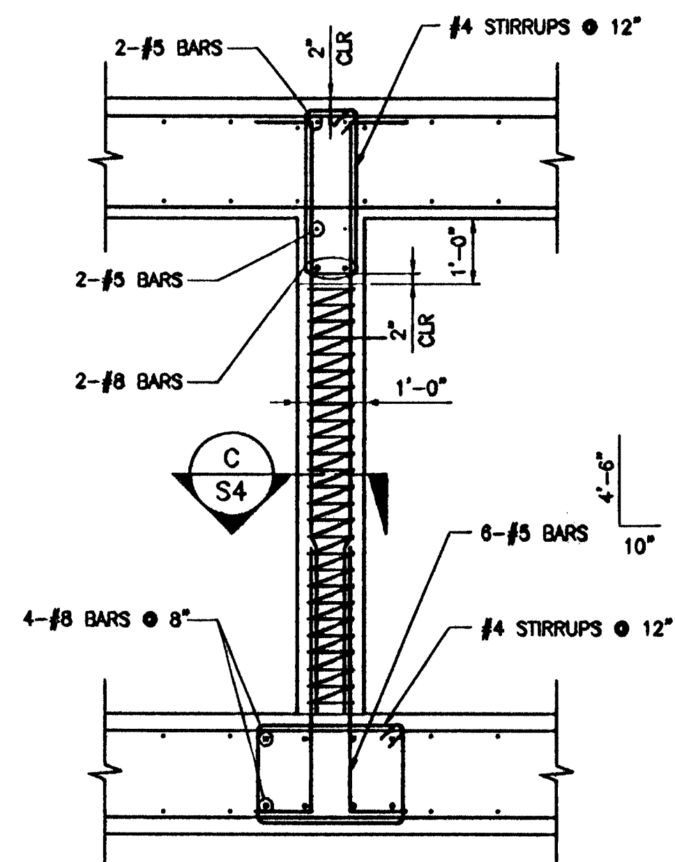
C SECTION SCALE: 1/2" = 1'-0"
