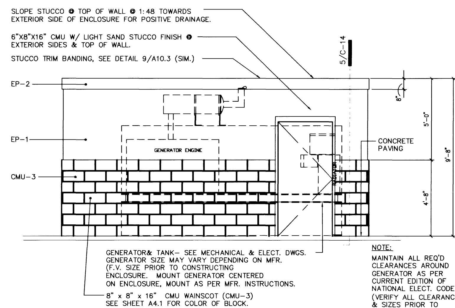
9A Generator Enclosure – South Elevation Scale: N.T.S. XXXX-XX AS2-11
