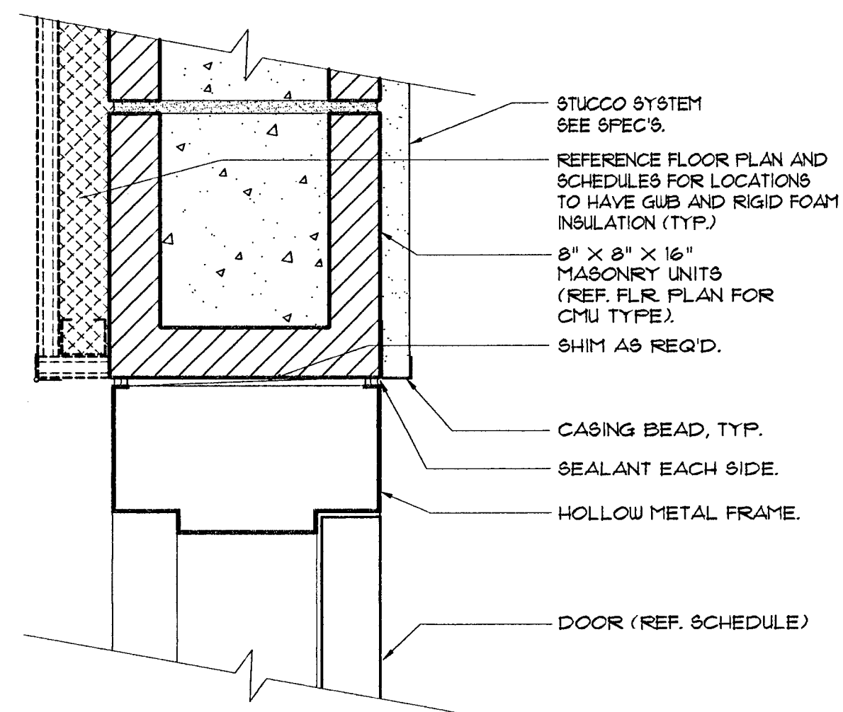
2 Head - Jamb @ Exterior Door Scale: 3\"/>
