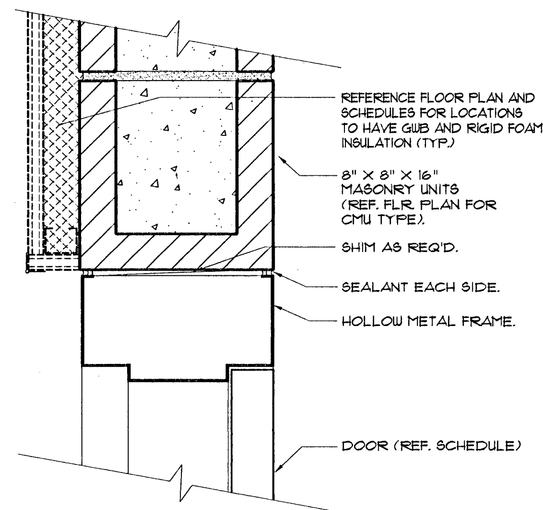
3 Interior Door Head / Jamb (Sim.) Scale: 3\"/>
