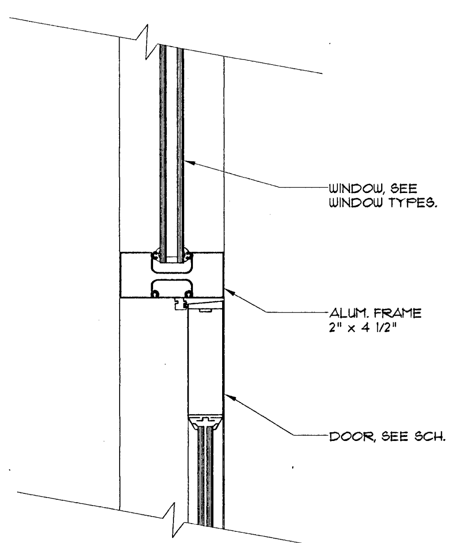
11 Head - Jamb Sim. Scale: 3\"/>
