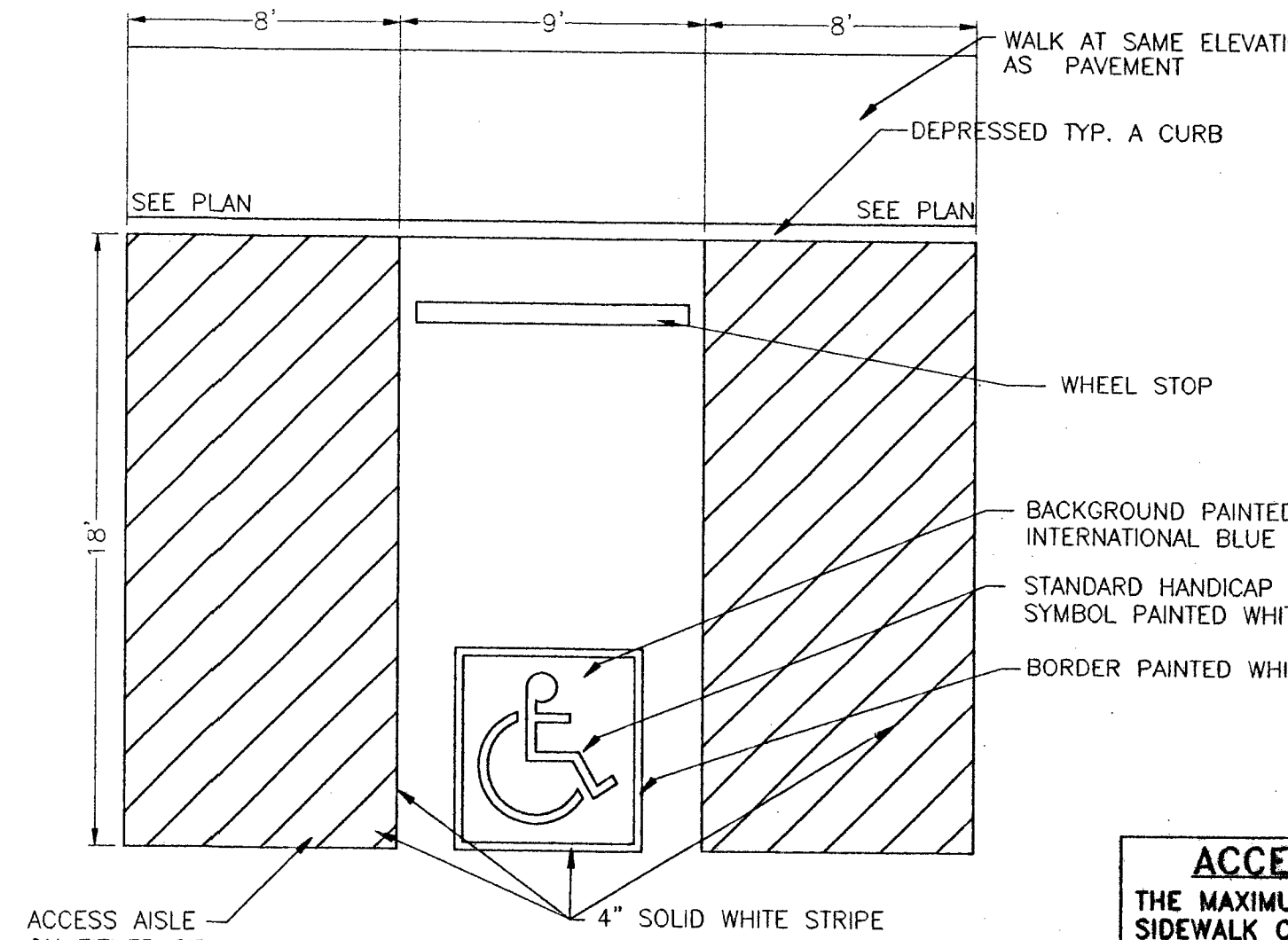
ACCESSIBLE PARKING STALL DETAIL (D) 1"=5'
